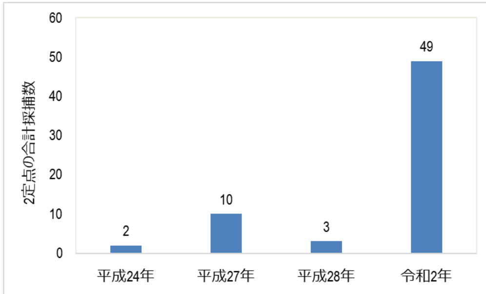
図2 小名浜定線における12月の合計採捕数（沿岸2定点のみ）
