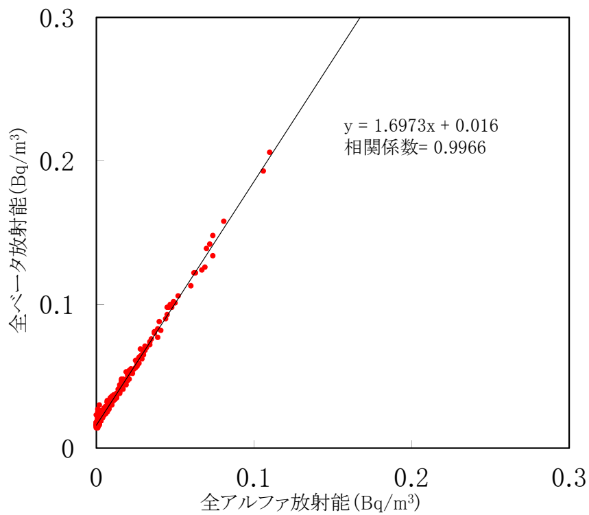
大気浮遊じんの全アルファ・全ベータ放射能の相関図 (MP-8) (令和2年7月～9月)
