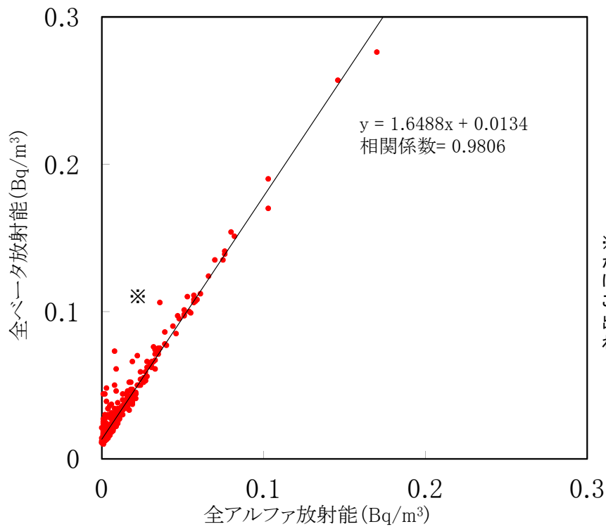
大気浮遊じんの全アルファ・全ベータ放射能の相関図 (MP-3) (令和2年7月～9月)
