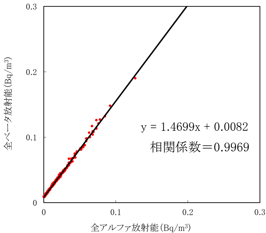
大気浮遊じんの全アルファ・全ベータ放射能の相関図 (MP-7) (令和2年7月～9月)
