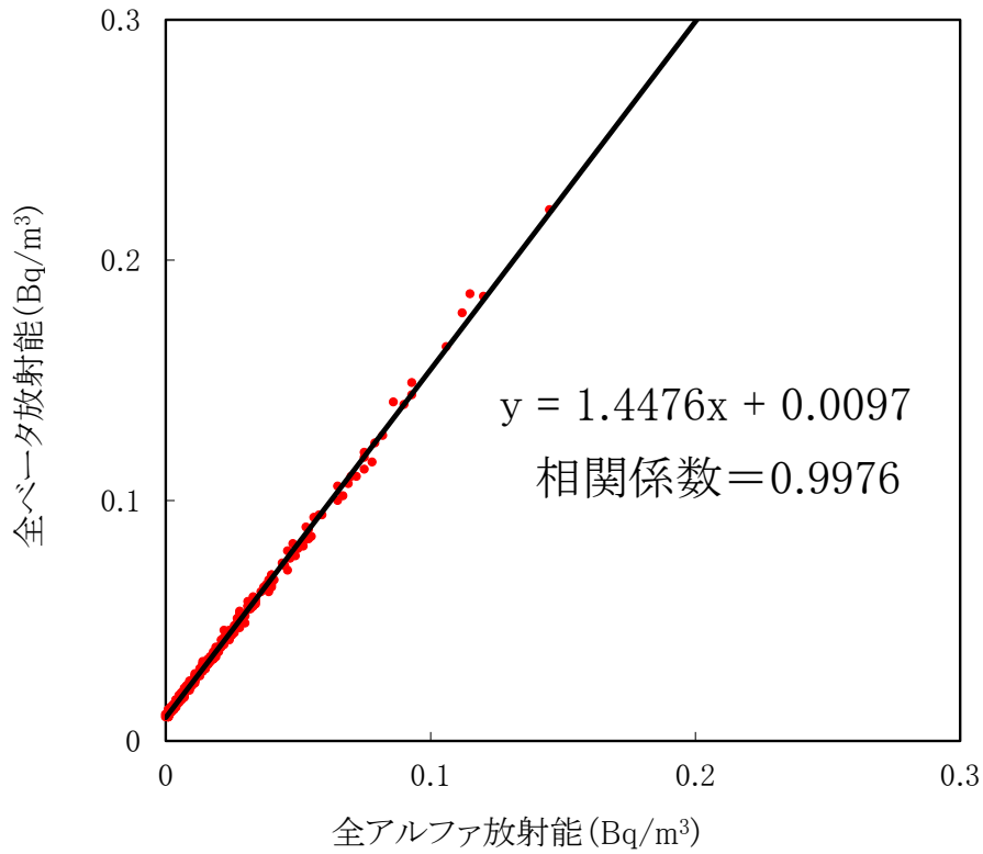
大気浮遊じんの全アルファ・全ベータ放射能の相関図 (MP-1) (令和2年7月～9月)
