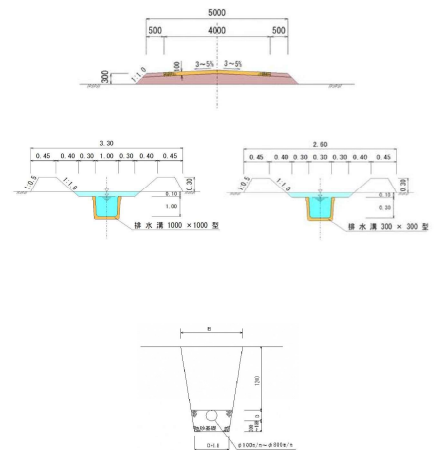
標準構造図
