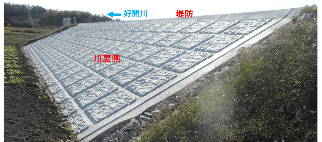
川裏側 コンクリート張ブロック完了 (6月末)
