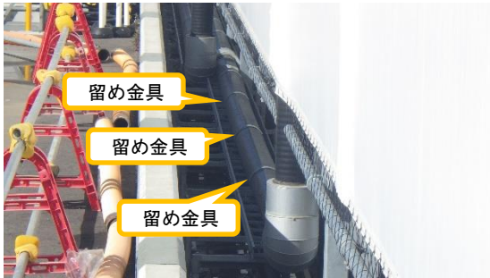
(写真1-2) G1南タンクエリア南側の配管の留め金具設置状況
