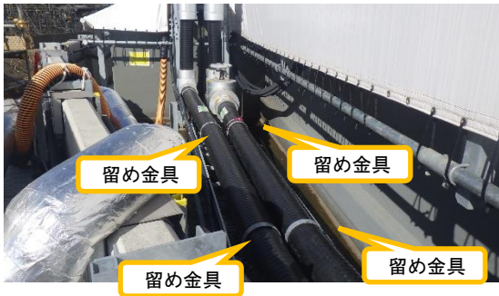
(写真1-3) G1南タンクエリア南西側の配管の留め金具設置状況
