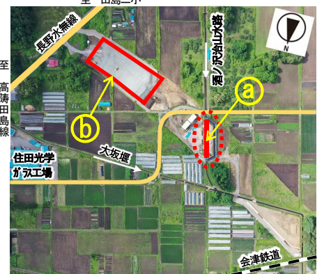
【写真1】工事状況全景写真
