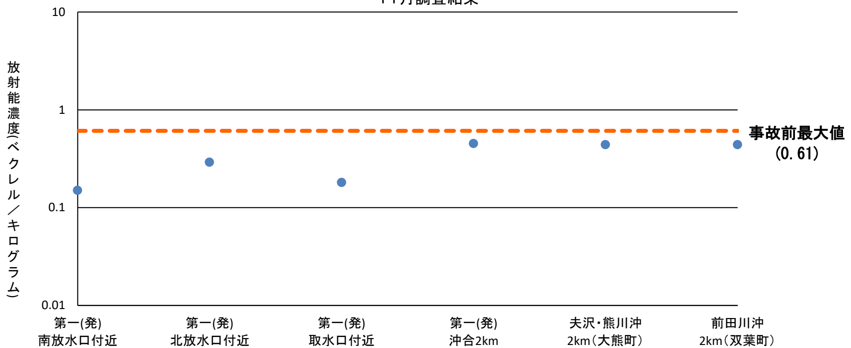
海底土中のプルトニウム濃度 (Pu-238+Pu-239+Pu-240) 11月調査結果
