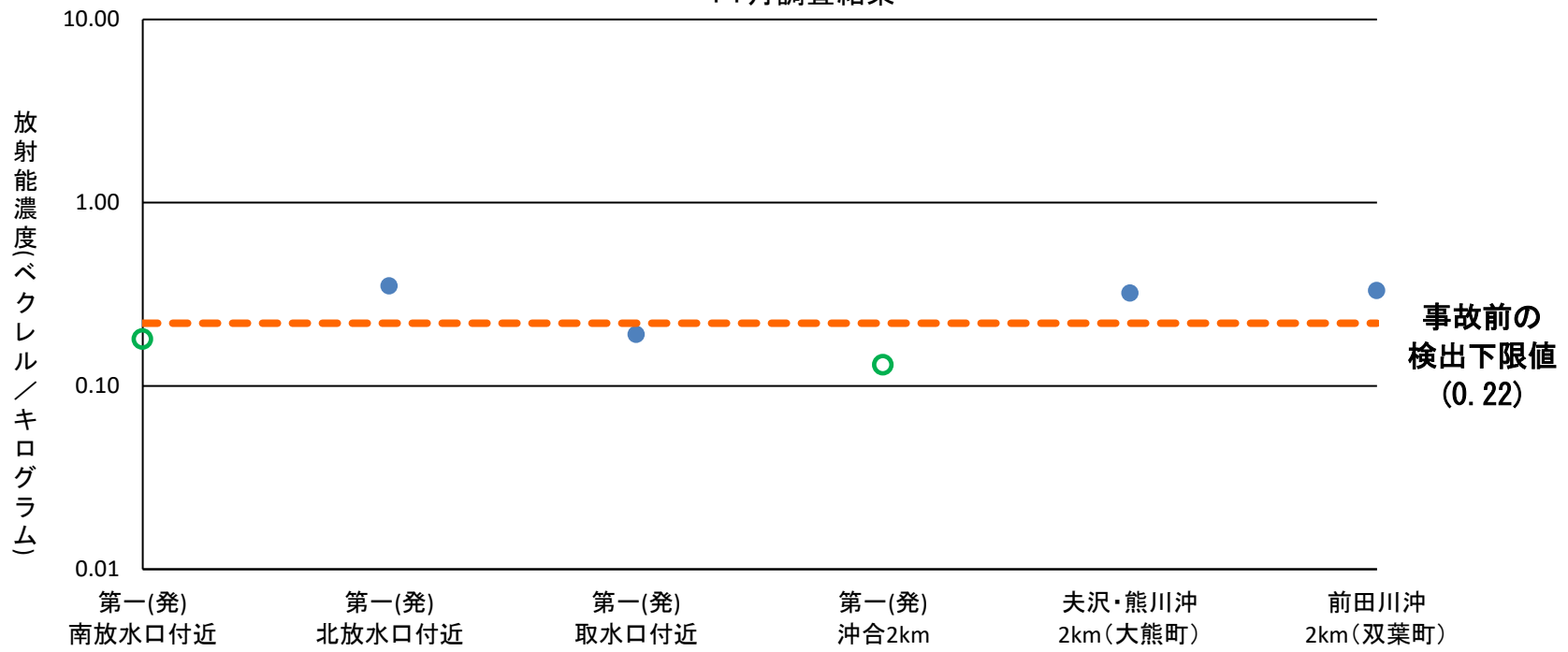
海底土中の放射性ストロンチウム濃度 (Sr-90) 11月調査結果
