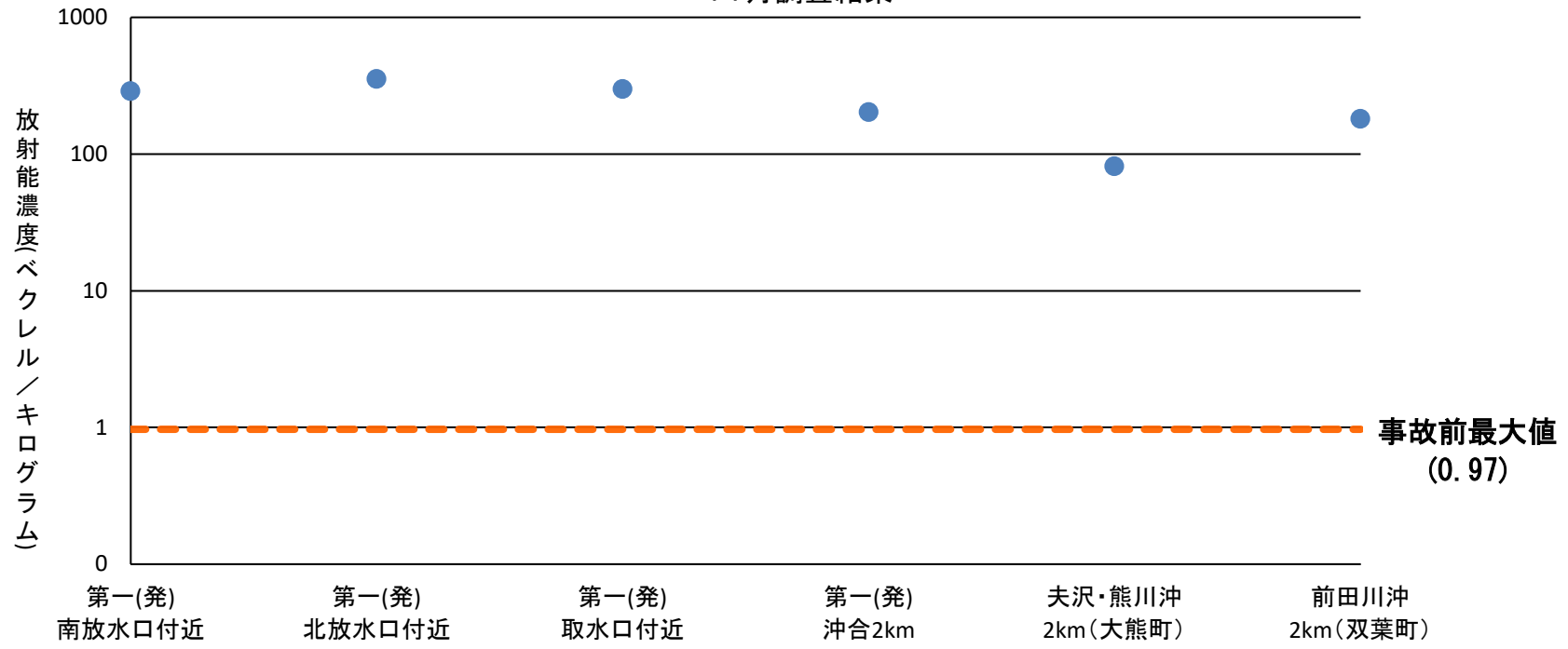
海底土中の放射性セシウム濃度 (Cs-134+Cs-137) 11月調査結果
