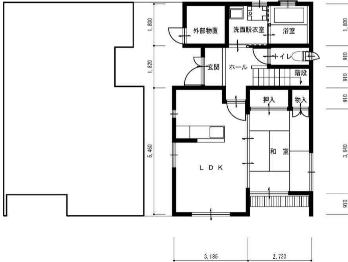
1階平面図 (3LDK)
