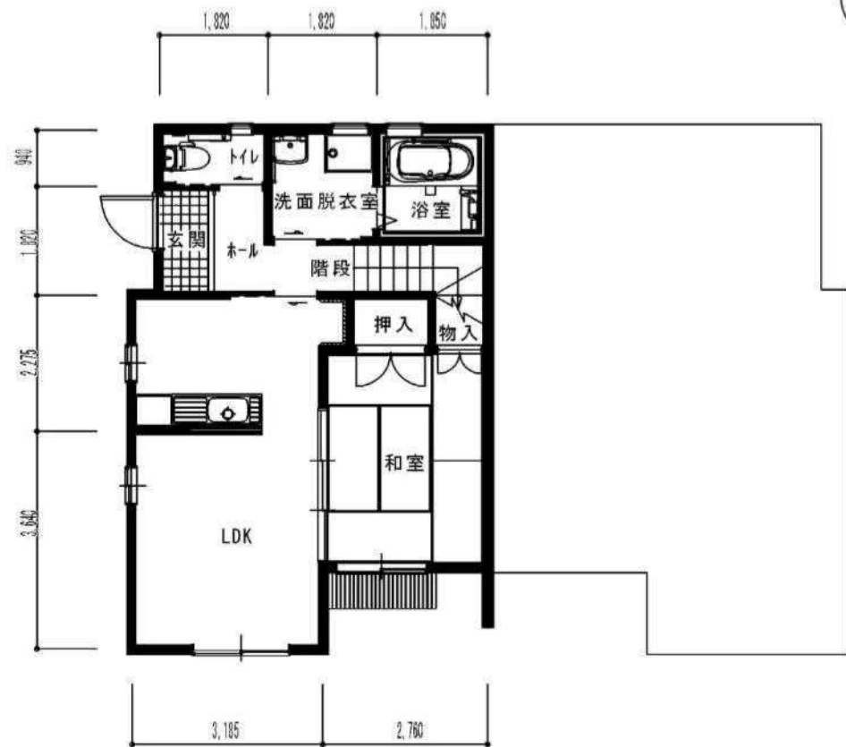
1階平面図
