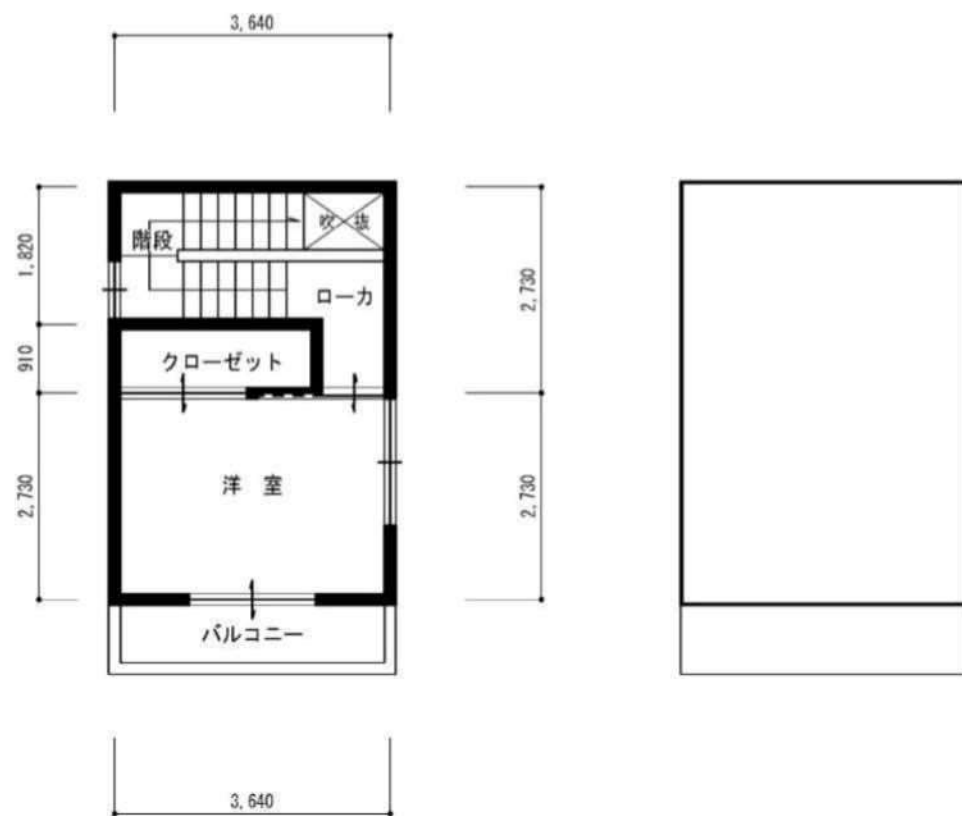
2階平面図 (2LDK)
