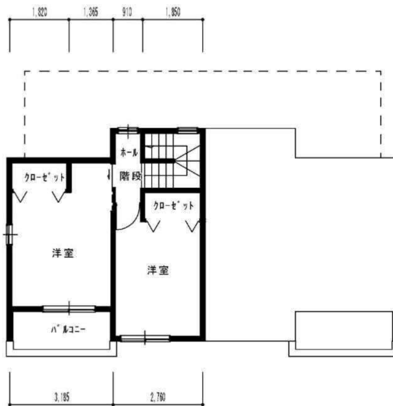
2階平面図
