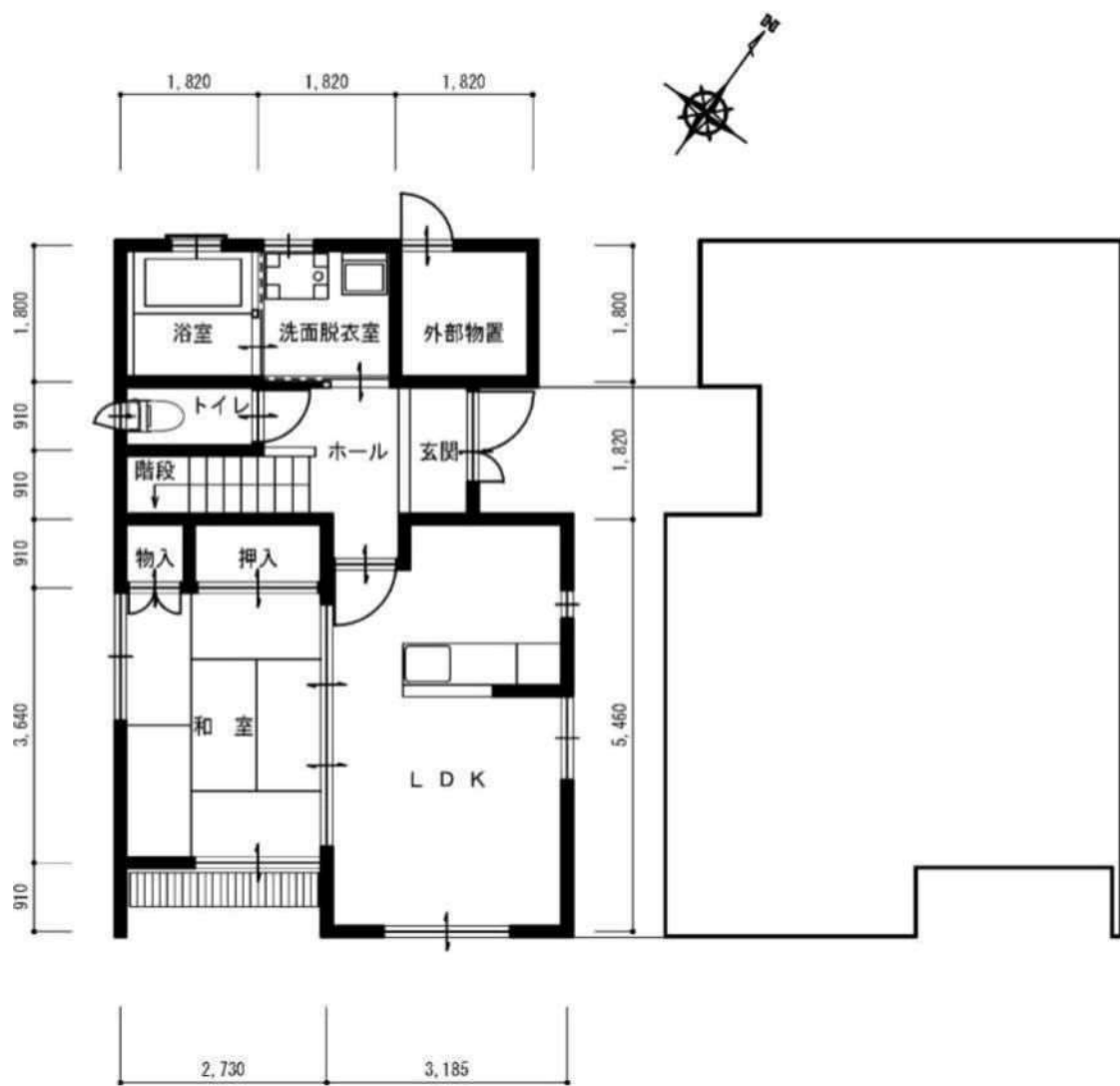
1階平面図 (2LDK)
