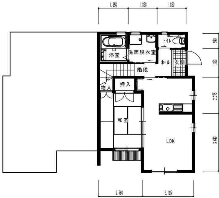
1階平面図
