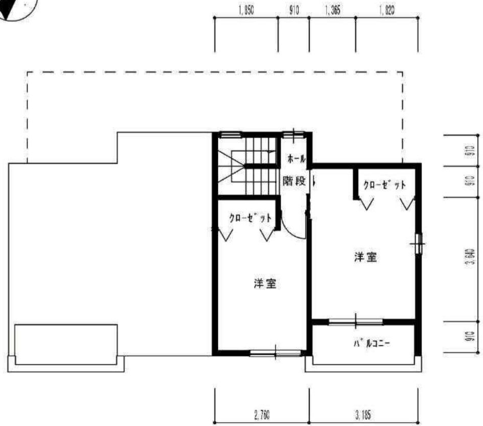
2階平面図
