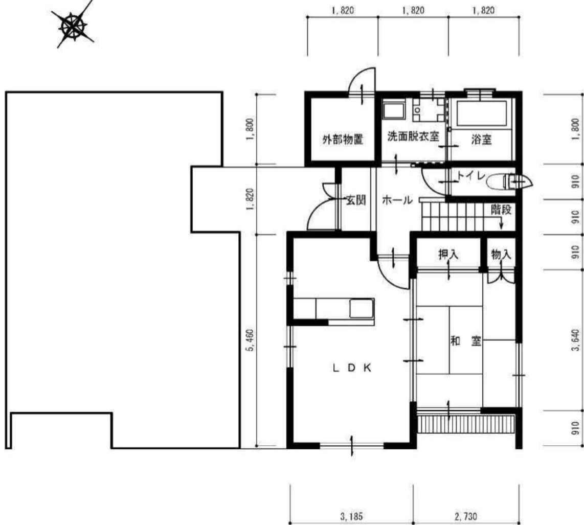
1階平面図 (2LDK)
