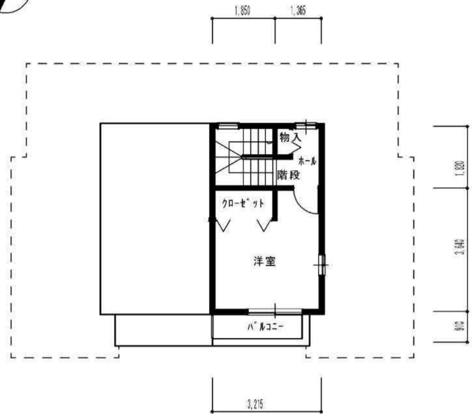
2階平面図
