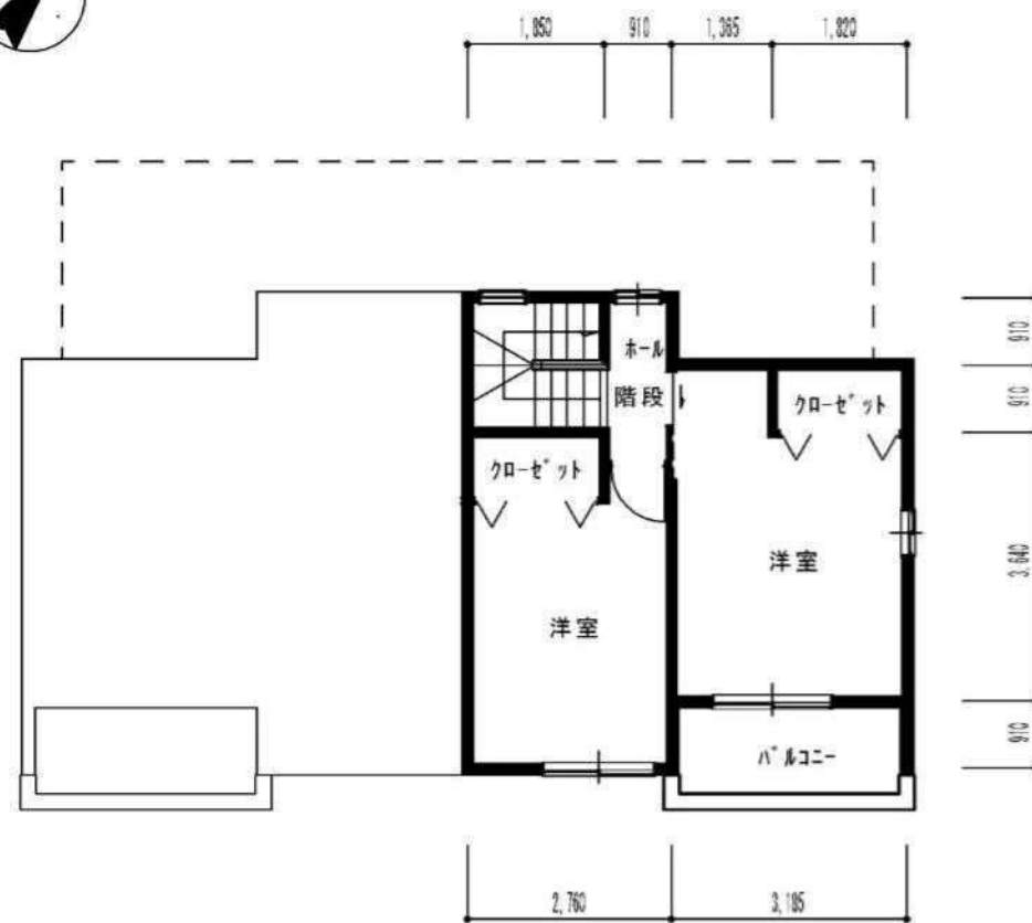
2階平面図
