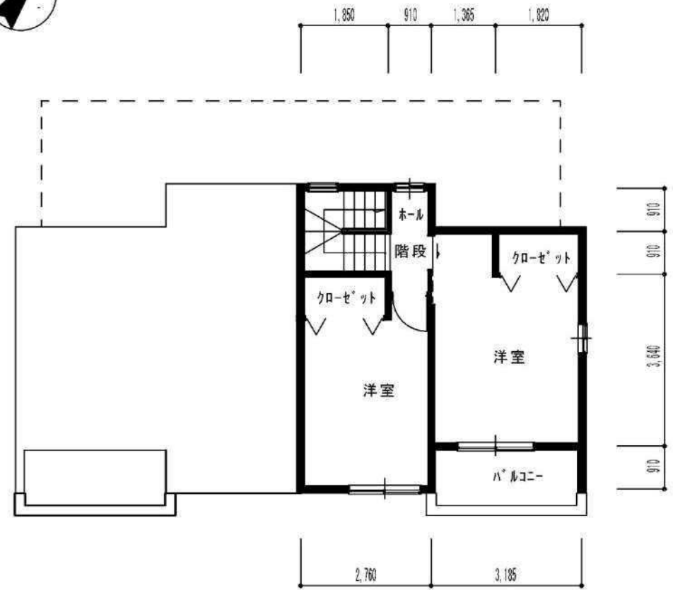
2階平面図
