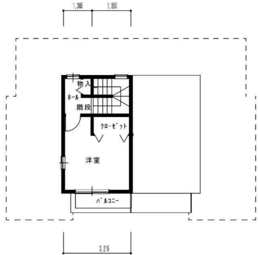
2階平面図
