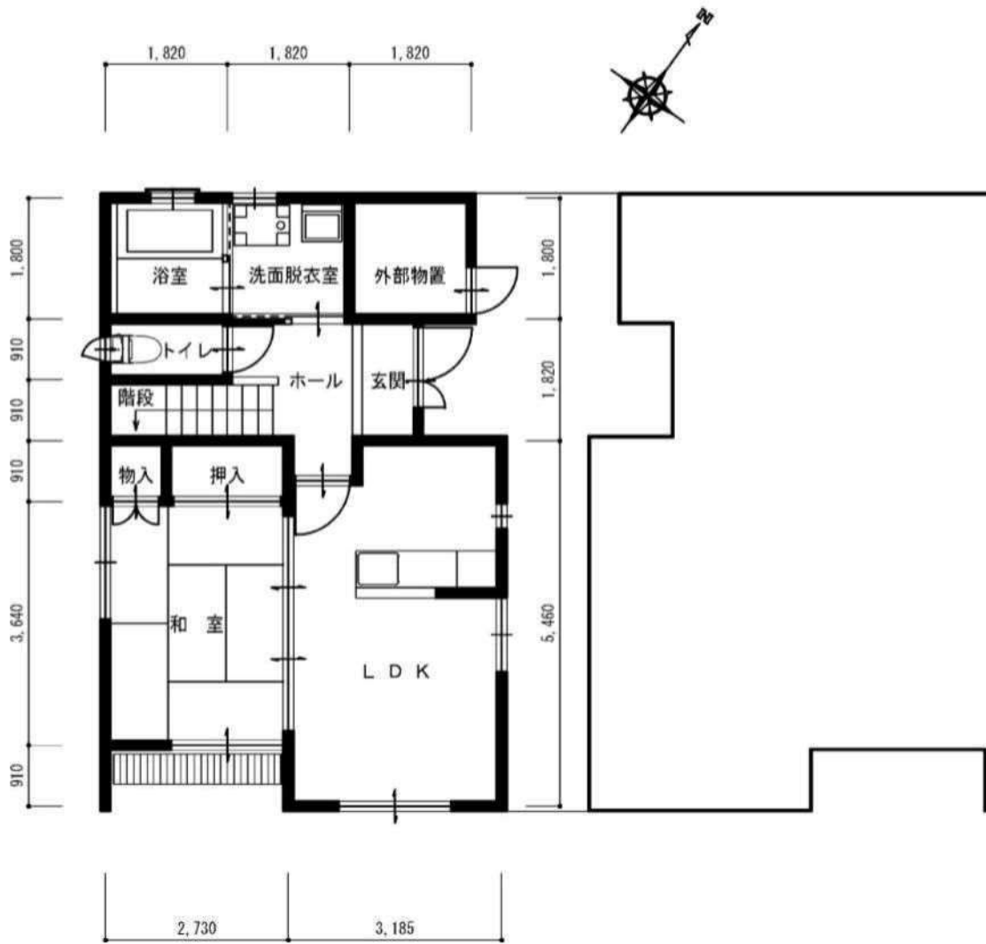
1階平面図 (3LDK)
