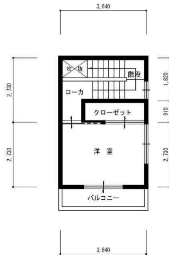
2階平面図 (2LDK)
