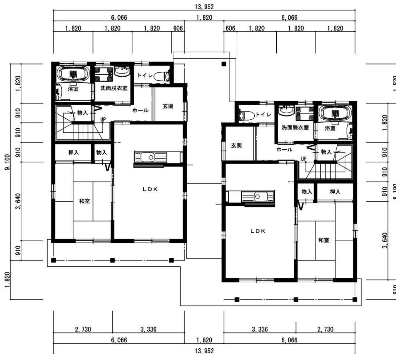
1階平面図
