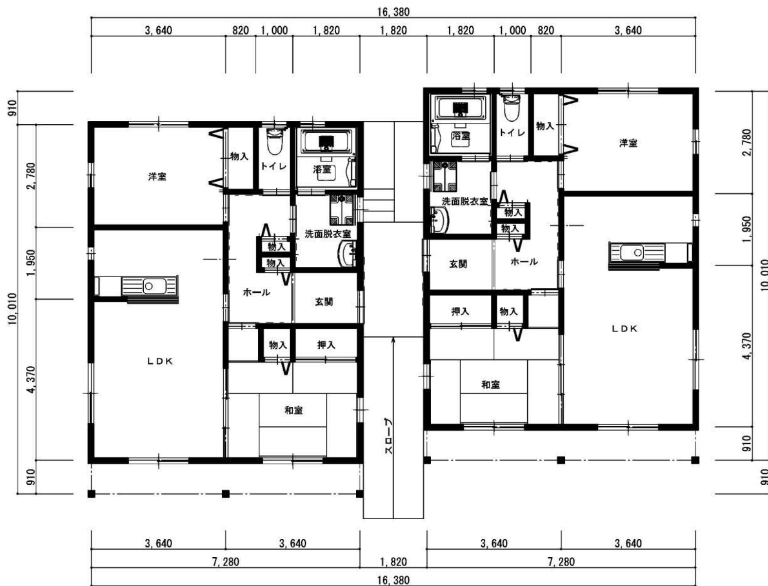
1階平面図
