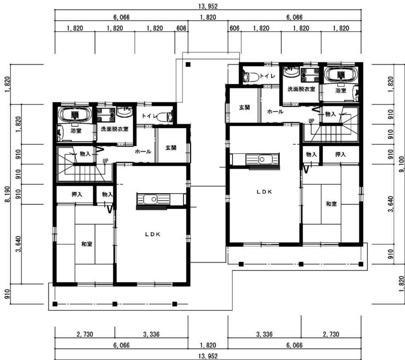
1階平面図
