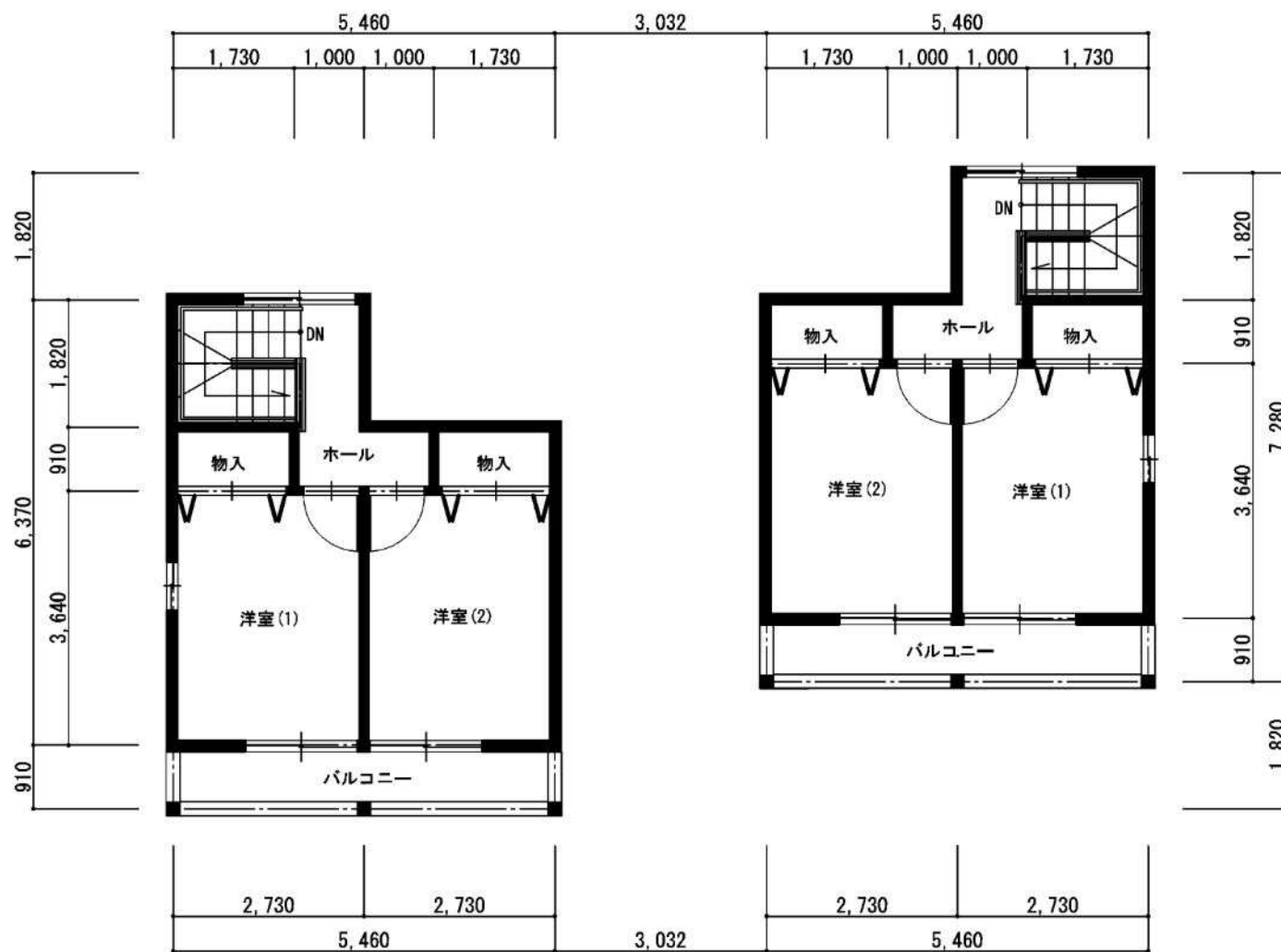
2階平面図
