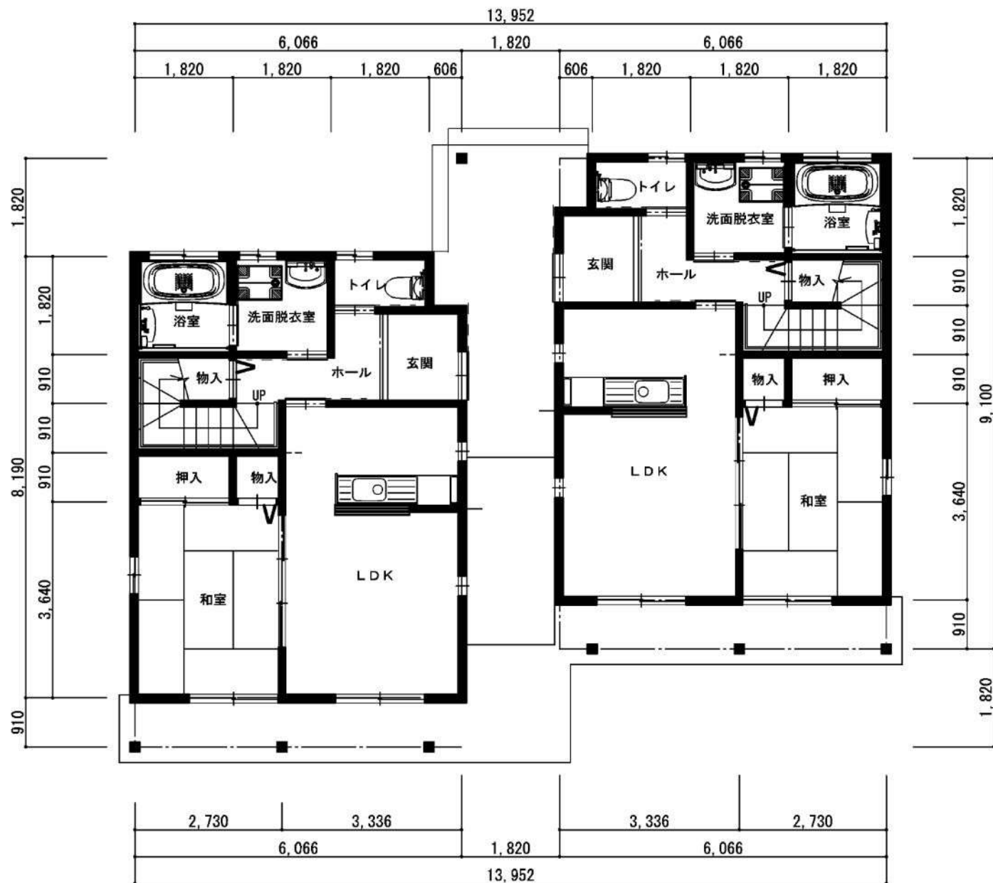
1階平面図
