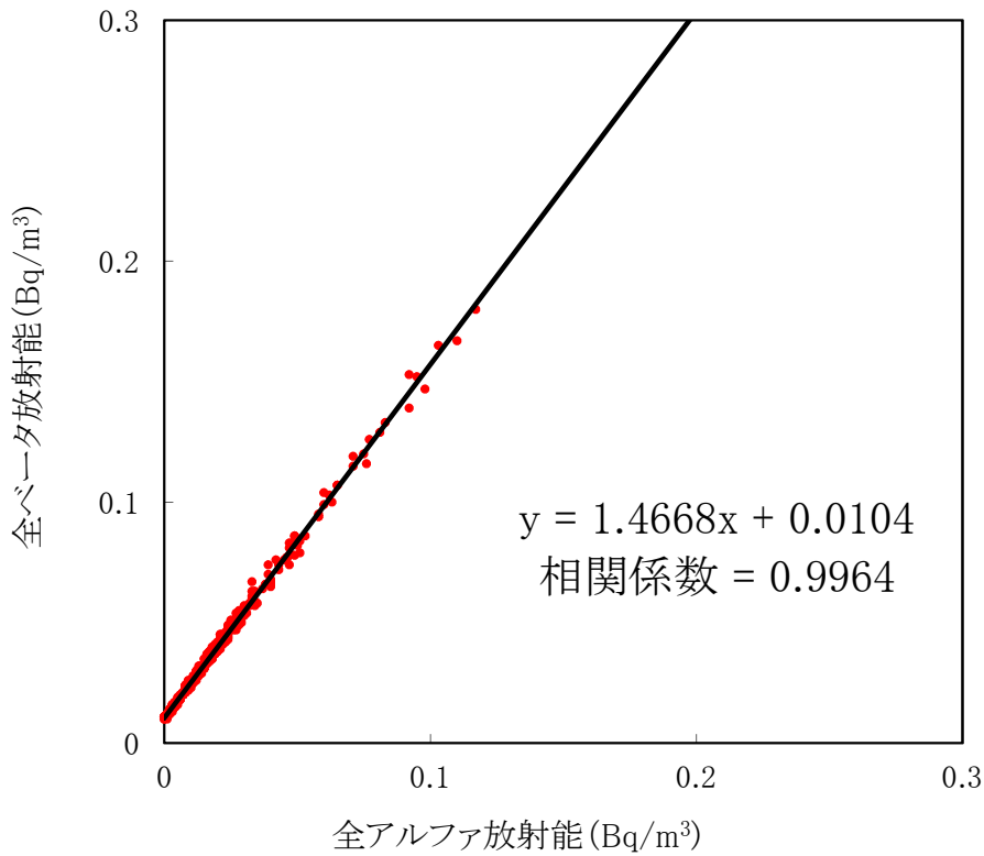
大気浮遊じんの全アルファ・全ベータ放射能の相関図 (MP-1) (令和元年7月～9月)
