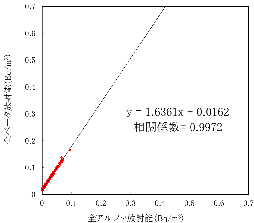
大気浮遊じんの全アルファ・全ベータ放射能の相関図 (MP-8) (令和元年7月～令和元年9月)
