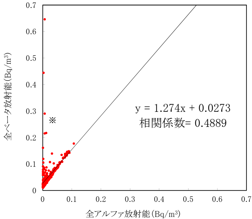
大気浮遊じんの全アルファ・全ベータ放射能の相関図 (MP-3) (令和元年7月～令和元年9月)
