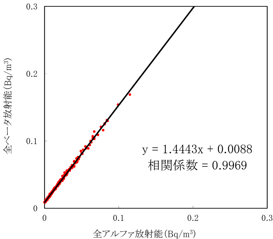
大気浮遊じんの全アルファ・全ベータ放射能の相関図 (MP-7) (令和元年7月～9月)
