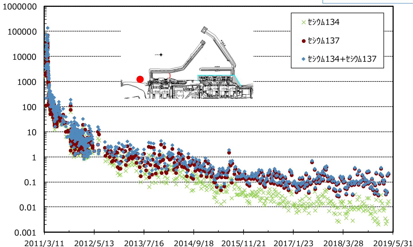
(ベクレル/リットル) 福島第一 5,6号機放水口北側 (T-1) 海水セシウム濃度
