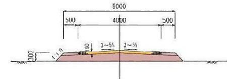
標準断面図 (小用水路)
