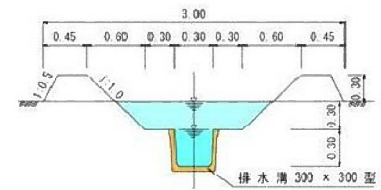
標準断面図 (小排水路)
