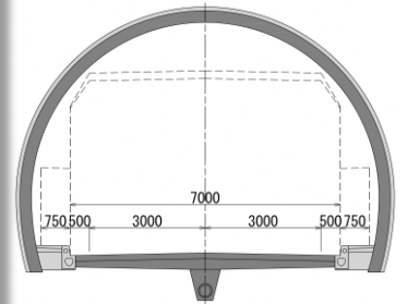
トンネル断面図
