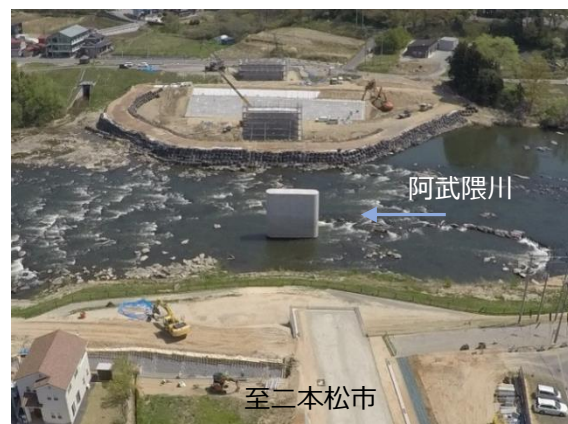
二本松金屋線 上ノ橋工区（本宮市仁井田）
