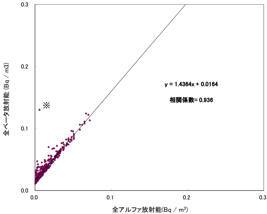
大気浮遊じんの全アルファ・全ベータ放射能の相関図 (MP-3) (平成29年10~12月)
