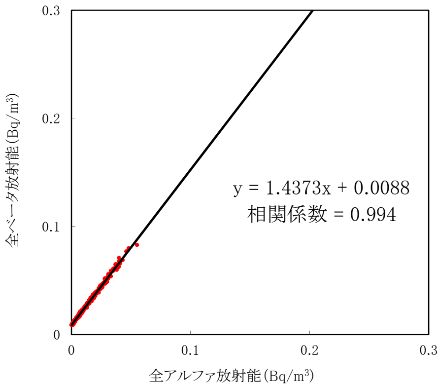
大気浮遊じんの全アルファ・全ベータ放射能の相関図 (MP-7) (平成29年10月～12月)
