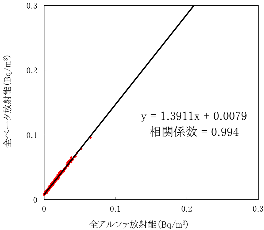
大気浮遊じんの全アルファ・全ベータ放射能の相関図 (MP-1) (平成29年10月～12月)
