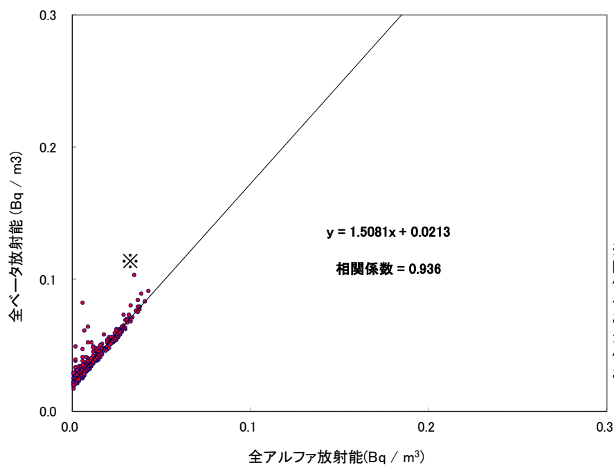
大気浮遊じんの全アルファ・全ベータ放射能の相関図 (MP-8) (平成29年10~12月)
