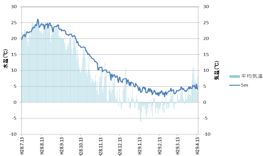
図 9 平成 28 年度における猪苗代湖長瀬川河口沖 300m の水深 5m 日平均水温及び日平均気温の関係
