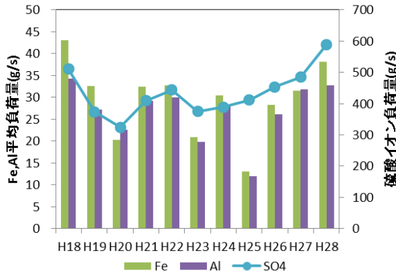
図 27 ② 硫黄川(高森川合流前)の酸性成分負荷量及び流量の経年変化
