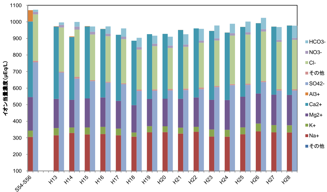
図 14 イオン当量濃度の経年変化 (3層平均)
