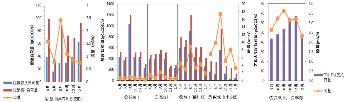
図 23 酸度負荷量及びアルカリ度負荷量の季節変動
