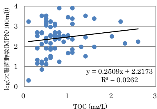
図25 TOCと大腸菌群数(2011～2016)
