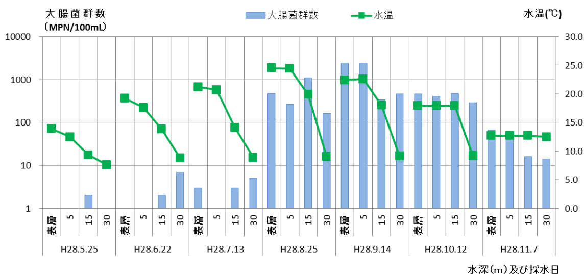
図4 湖心大腸菌群数と水温の推移
