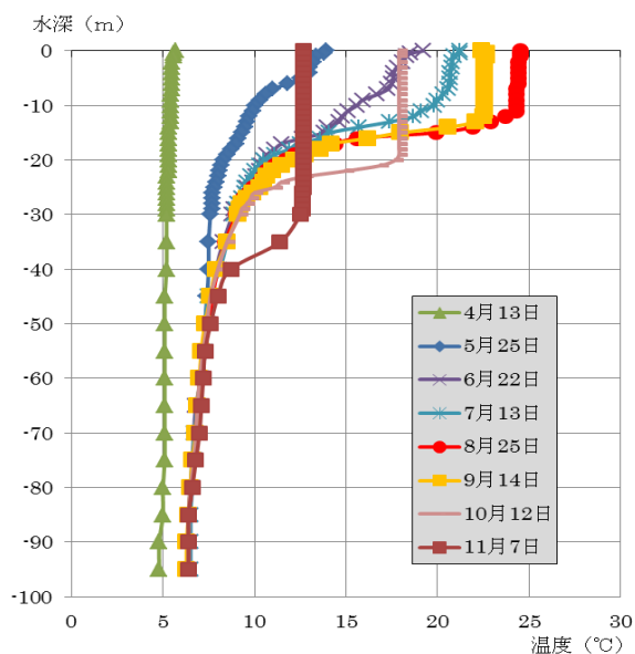
図 3 湖心の鉛直分布
