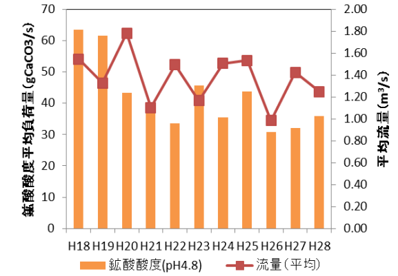
図 29 ④ 酸川(高森川合流前)の酸性成分負荷量及び流量の経年変化
