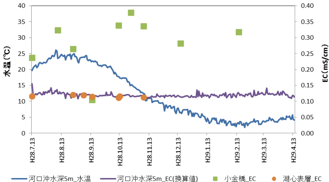
図 10 長瀬川河口沖 300m 地点（水深 5m）における水温及び EC の日平均値と、 小金橋及び湖心表層における EC の比較
