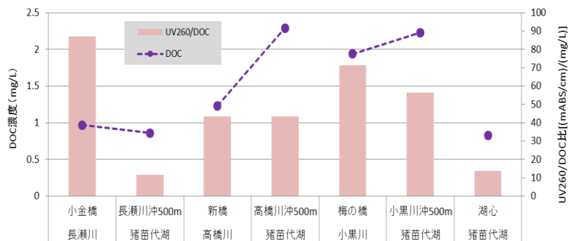
図5 UV260/DOC 比及び DOC 濃度
