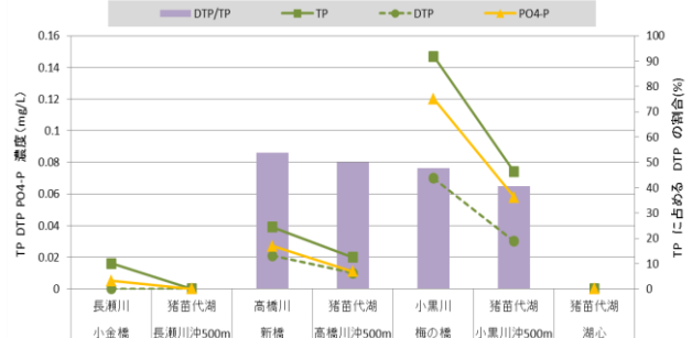
図4 T-P等の濃度及び溶存態の割合
