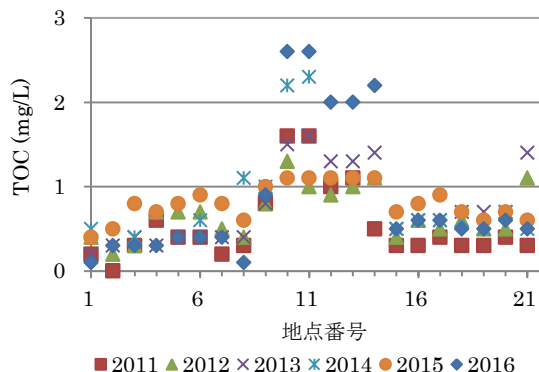
図 11 TOC
