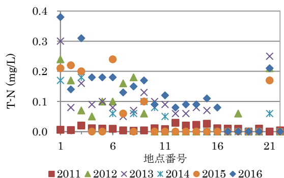
図 13 全窒素
