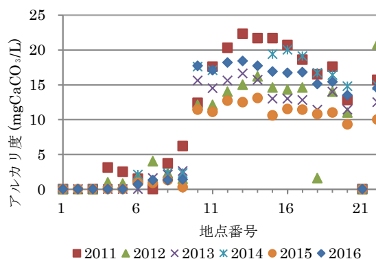
図 14 アルカリ度
