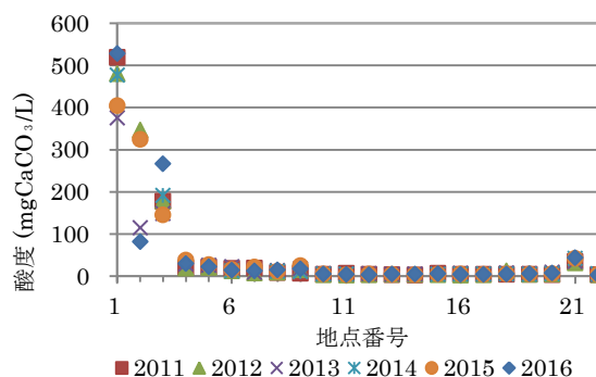
図 15 酸度
