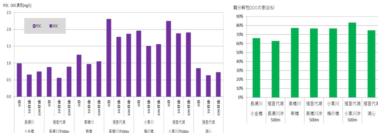
図 8 生分解試験 30 日後の難分解性 DOC の割合
