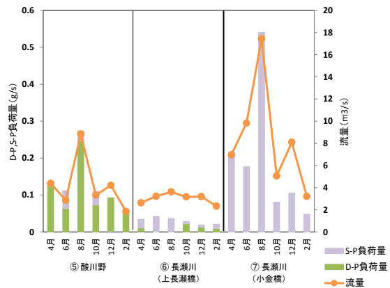
図 26 D-P 及び S-P 負荷量の季節変動
