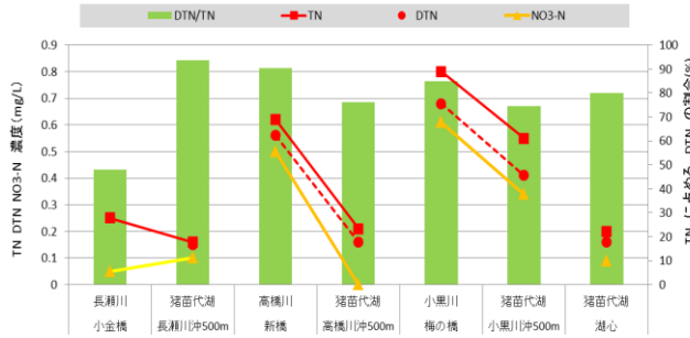
図3 T-N等の濃度及び溶存態の割合
