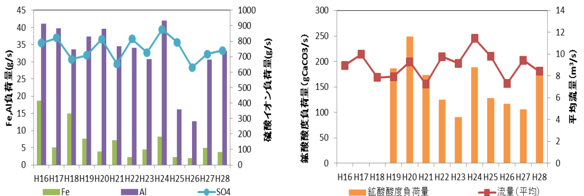
図32 ⑦ 長瀬川(小金橋)の酸性成分負荷量及びアルカリ度負荷量及び流量の経年変化
