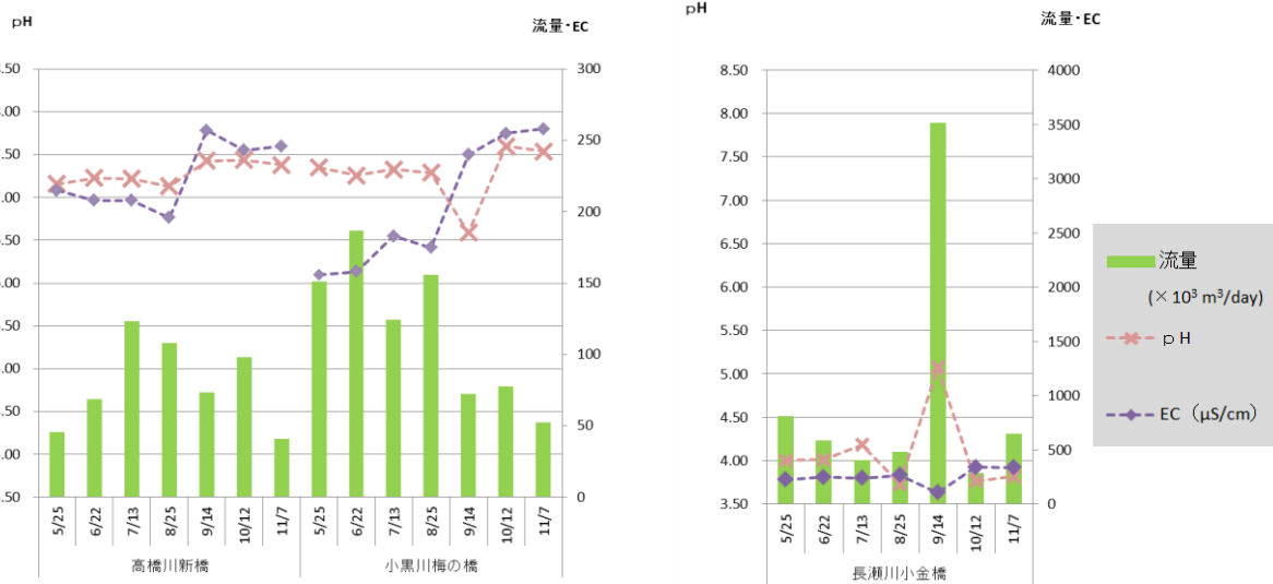
図 11 各河川の流量と pH 等の推移
