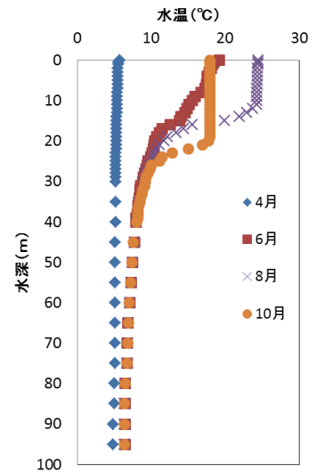
図 2 鉛直水温
