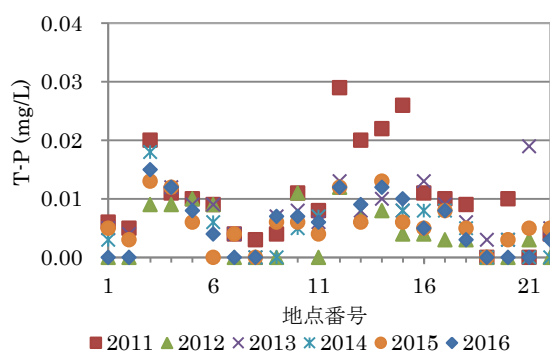
図 12 全リン
