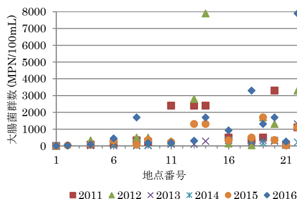
図 21 大腸菌群数
