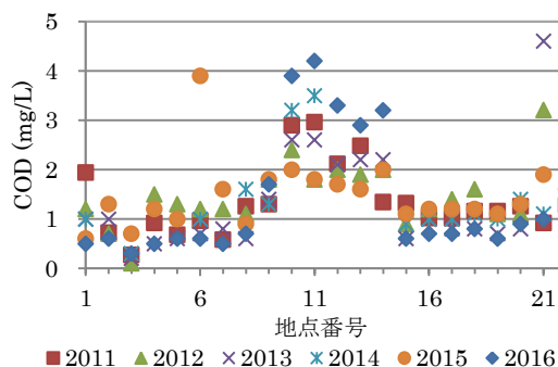
図 10 COD
