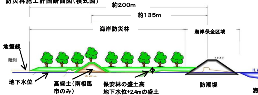
防災林施工計画断面図(模式図)
