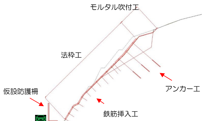
<復旧計画図>
