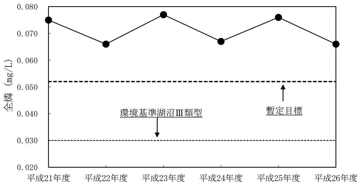
図3 千五沢ダム貯水池における全リンの経年変化（表層・年平均値） （全リン：環境基準Ⅲ類型 0.03mg/L）
