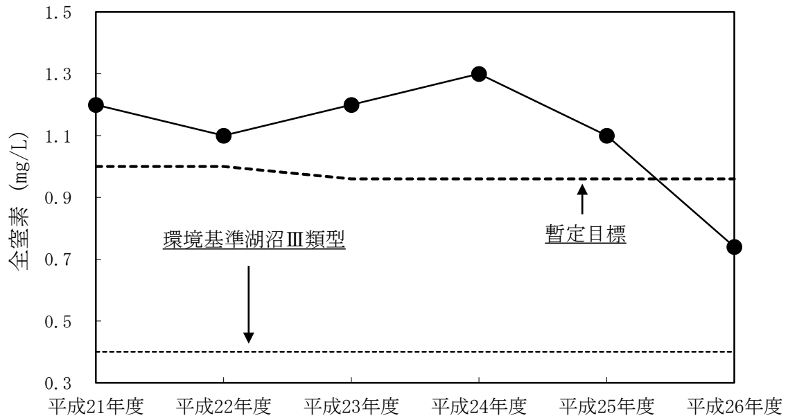
図2 千五沢ダム貯水池における全窒素の経年変化（表層・年平均値） （全窒素：環境基準Ⅲ類型 0.4mg/L）
