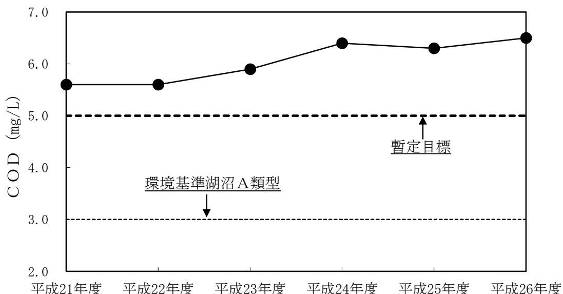
図1 千五沢ダム貯水池におけるCODの経年変化（全層・75%値）
