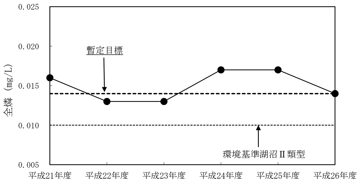
図5 東山ダム貯水池における全磷の経年変化（表層・年平均値）
