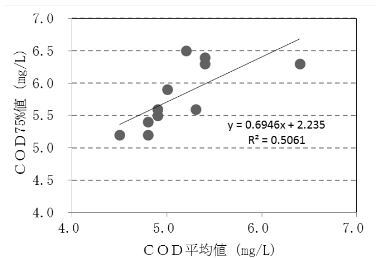
図4 千五沢ダム貯水池（ダムサイト）におけるCOD平均値と75%水質値の関係（過去10年間）
