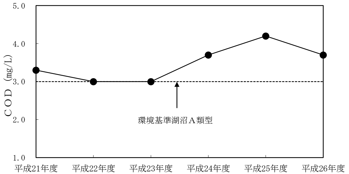
図6 東山ダム貯水池におけるCODの経年変化（全層・75%値） （COD：環境基準A類型 3mg/L）
