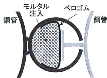
海側遮水壁の継手構造
