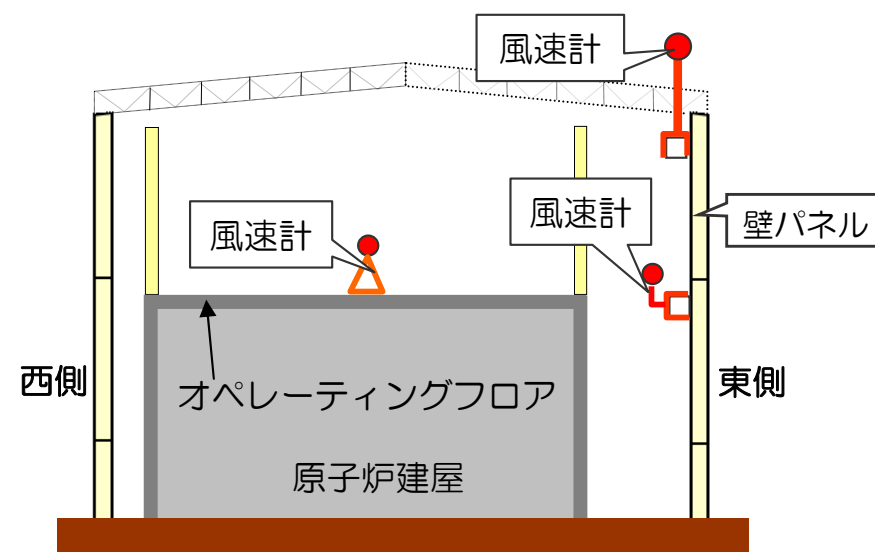
風速測定イメージ
