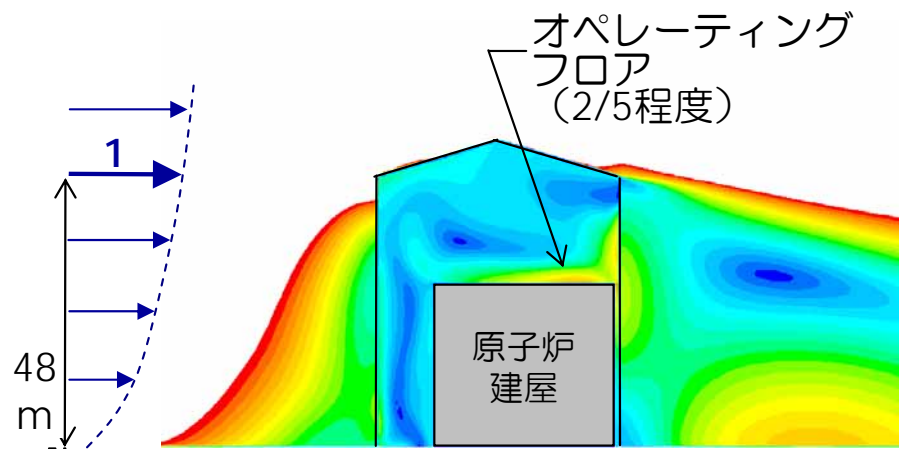
屋根パネル2枚外した状態（東風）
