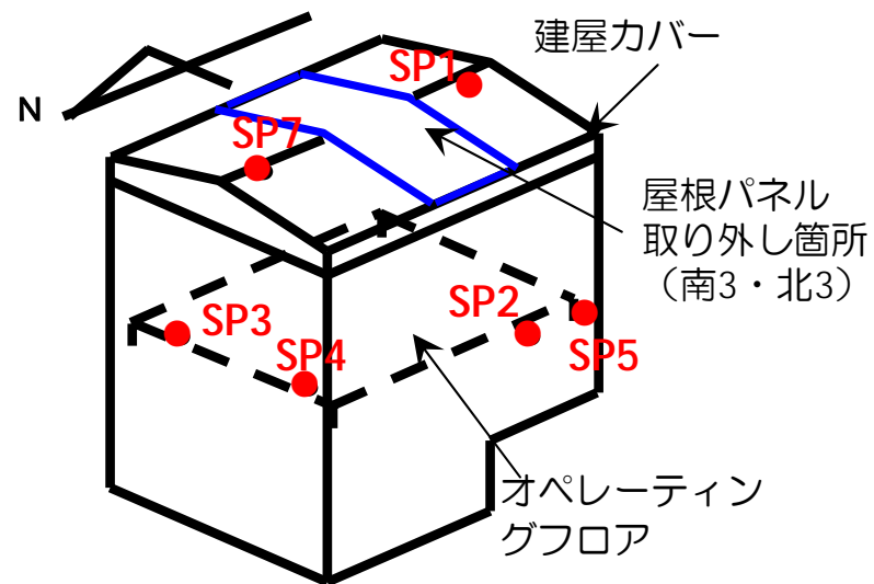
ダストモニタのサンプリング箇所
