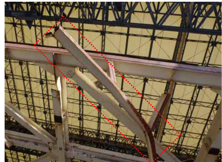
③ 7a通り付近 鉄骨損傷
