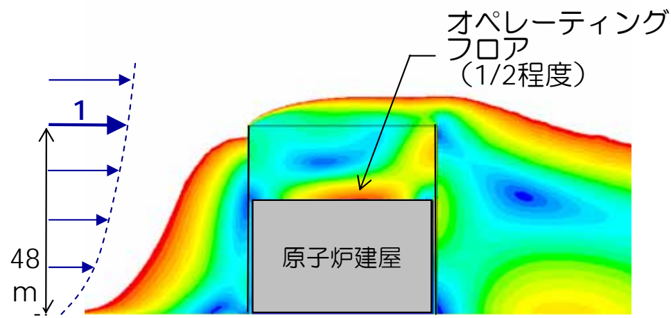
屋根パネル6枚外した状態（南風）
