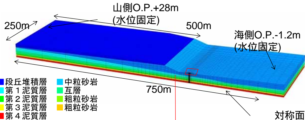
解析メッシュ図(1/2対称モデル)
