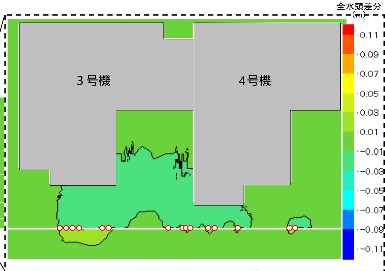
部分先行凍結前に対する凍結後の地下水位増減 (地下水位の差分コンター 3次元浸透流解析による)
