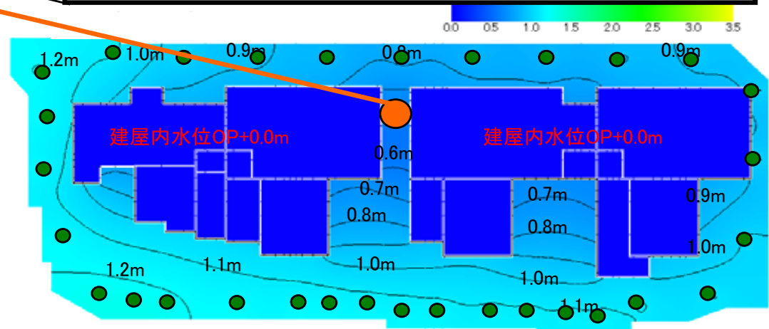
図 地下水位コンター（60ヶ月）
