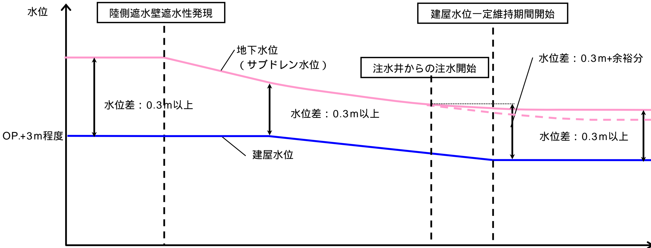
地下水位低下に伴う建屋内外の水位管理 (イメージ)
