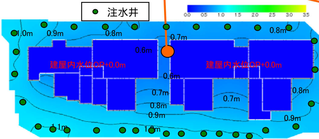
図 地下水位コンター（30ヶ月）
