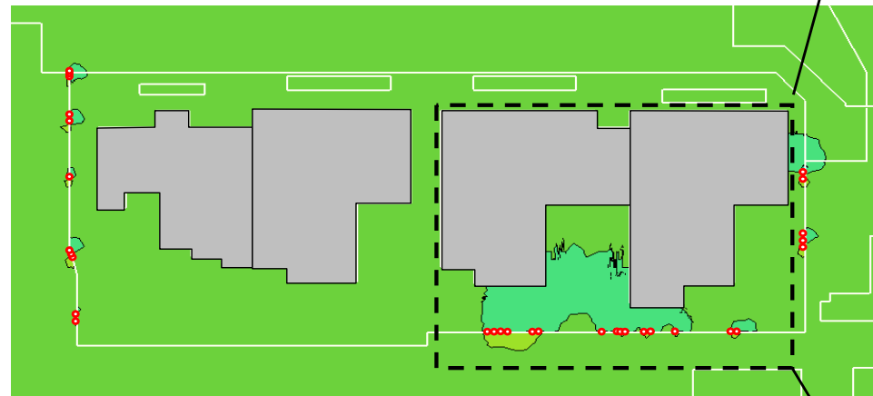
部分先行凍結前に対する凍結後の地下水位増減 (地下水位の差分コンター 3次元浸透流解析による)
