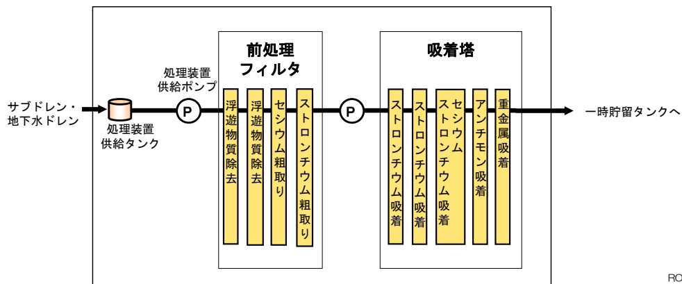
サブドレン浄化設備 系統概略図
