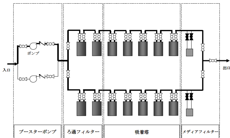
【参考】SARRY 系統概略図
