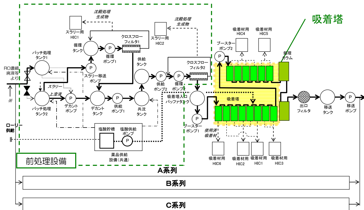
多核種除去設備 系統概略図
