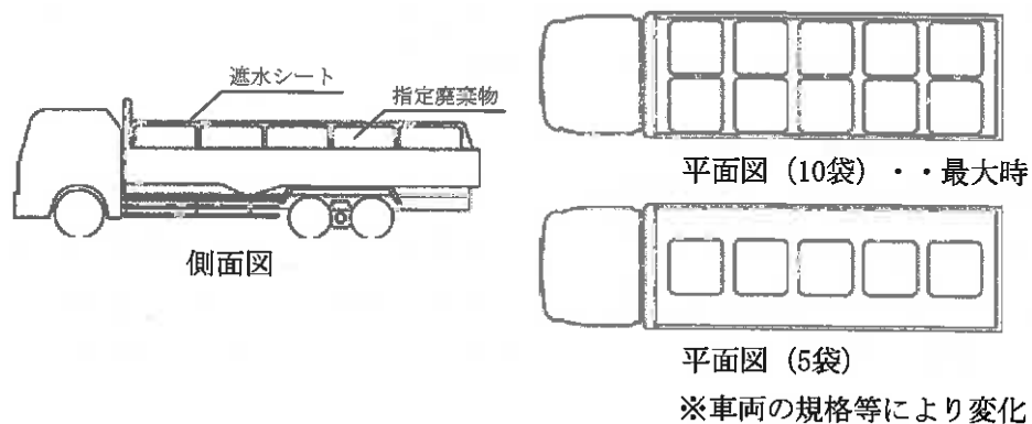
図4-3 荷姿の例 (10トントラックの場合)
