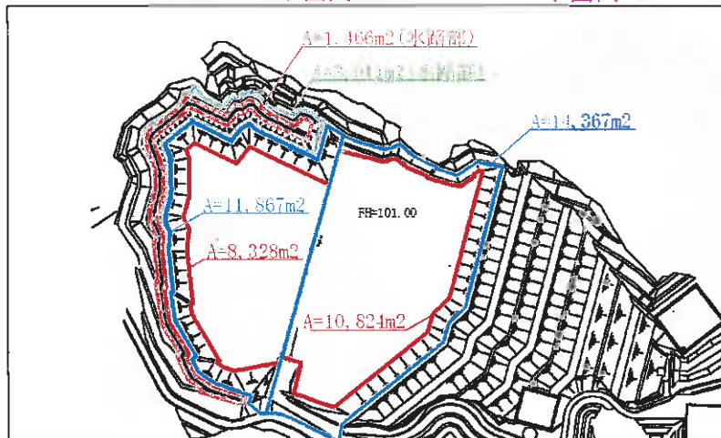
図 2-5(3) 埋立容量計算の根拠図(7~9 段目)
