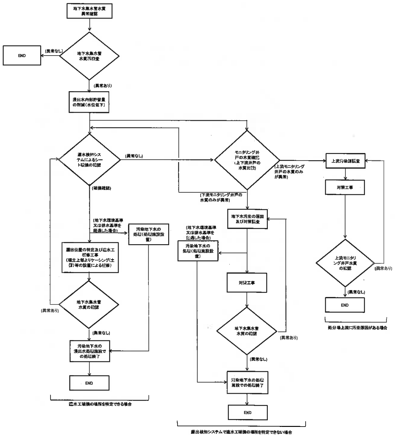
図 3-5(1) 地下水水質に異常が発生した場合の対応 (含む遮水シートの破損が確認された場合)
