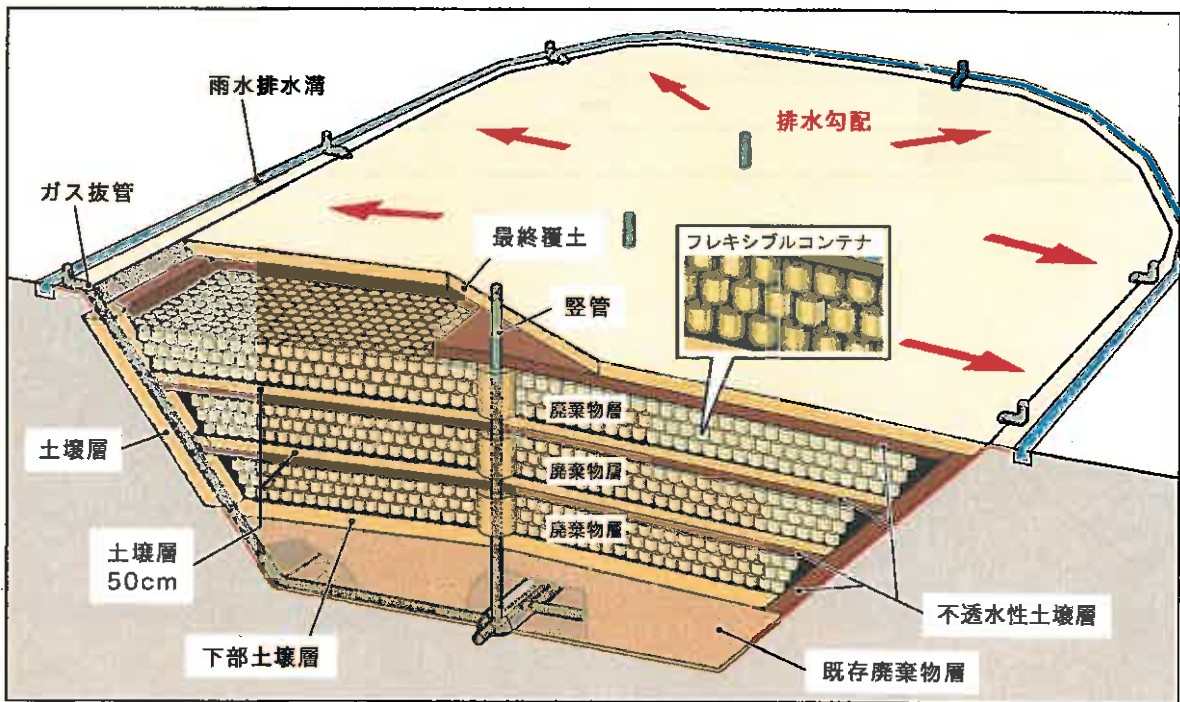
セメント固型化しない廃棄物の埋立層
