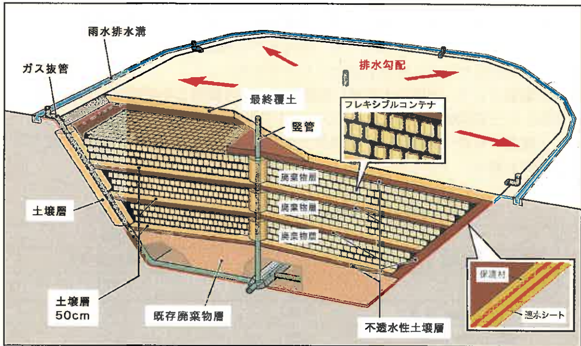
セメント固型化した廃棄物の埋立層
