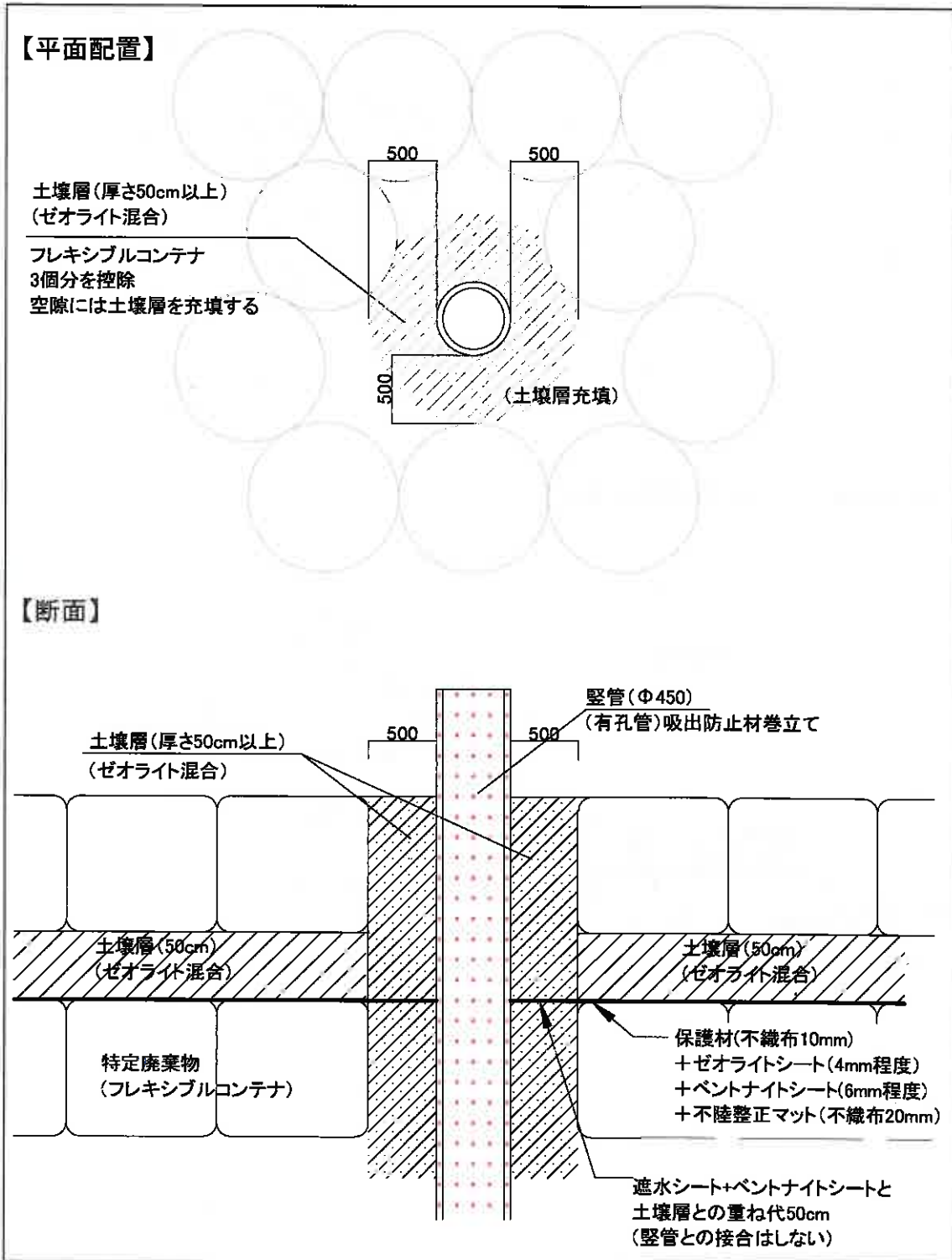
図 2-15 豎管の標準構造
