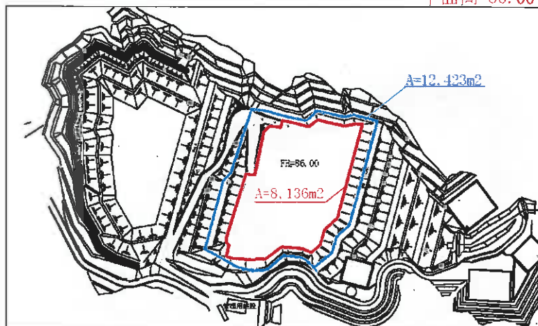
図 2-5(2) 埋立容量計算の根拠図 (4~6 段目)
