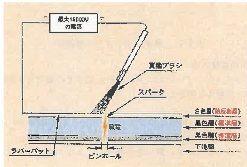
図 1-8 遮水シートのスパーク検査
