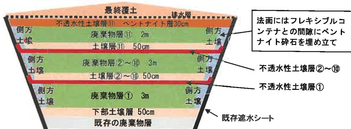
図2-7(2) セメント固型化しない廃棄物の埋立層
