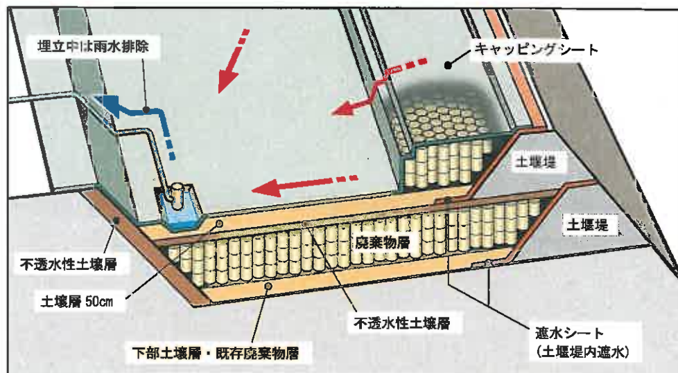
図 2-9(2) 埋立区画の排水勾配 (縦断図)
