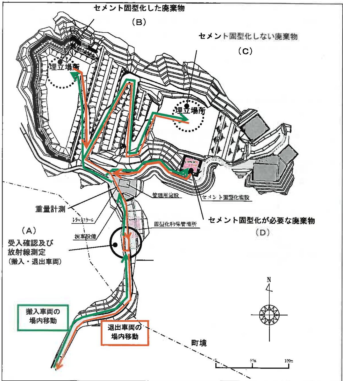
図 2-2(1) 搬入車両の場内移動
