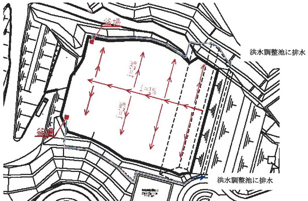
図 2-9(1) 埋立区画の排水勾配 (平面図)
