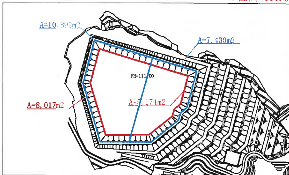
図 2-5(4) 埋立容量計算の根拠図(10~11 段目)
