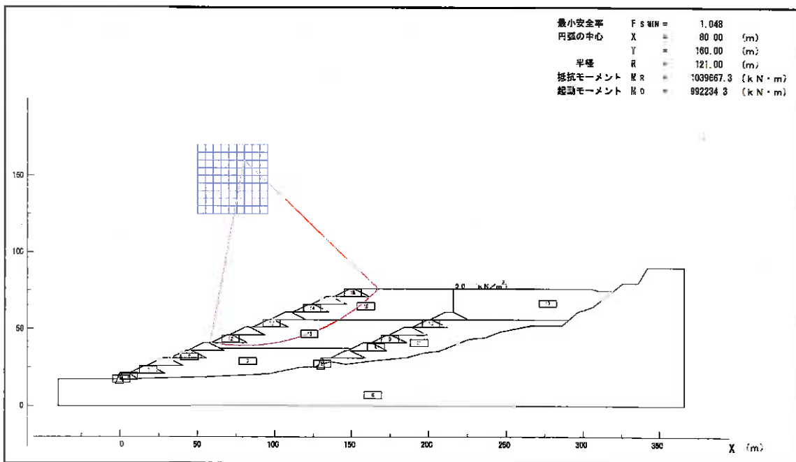
図 2-6 (1) 浅いすべり面（セメント固型化しない廃棄物層）
