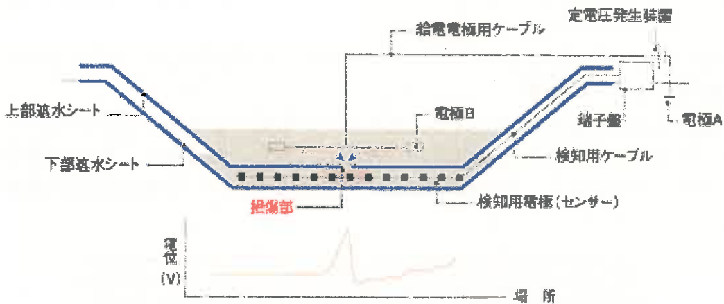
図 1-7 漏水検知システム概要図
