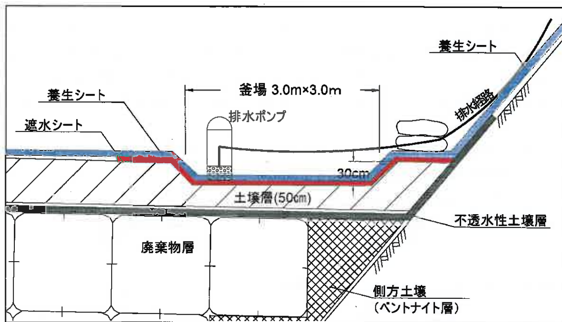
図 2-12 釜場の設置
