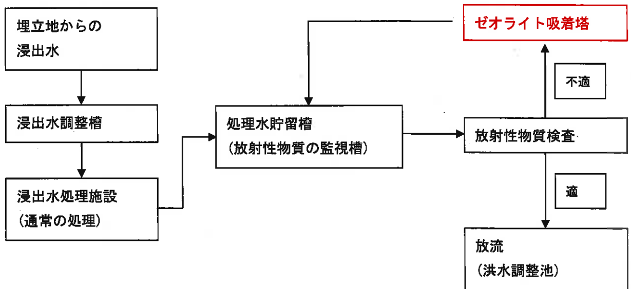
図 2-17 浸出水処理施設改良後の処理フロー
