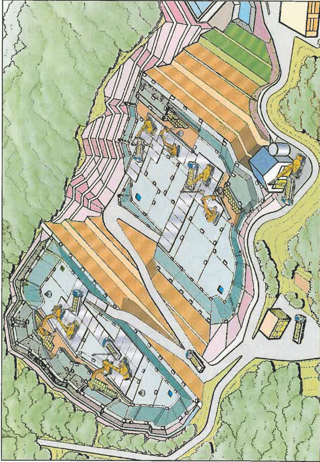
图 2-1(2) 埋立作業図(例) (上段側 9 段目、下流側 6 段目)
