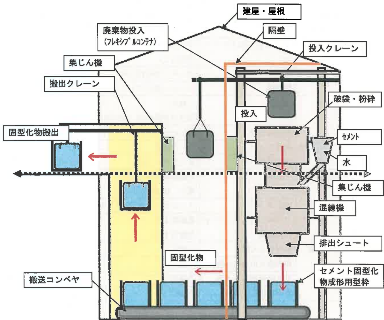
図 2-3(1) セメント固型化施設のイメージ図
