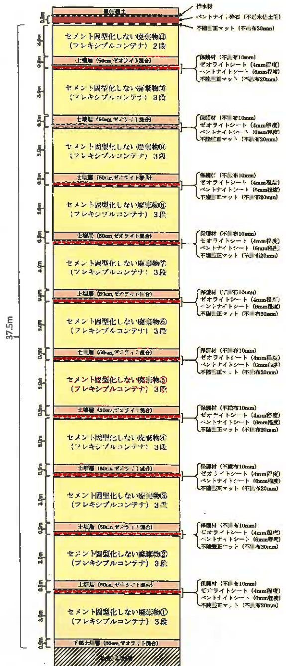
図 2-8(1) 埋立廃棄物層の構成
