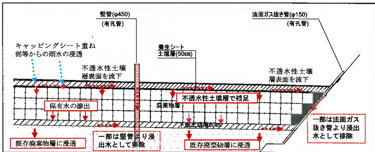
図 2-13 廃棄物層からの浸出水排除方法
