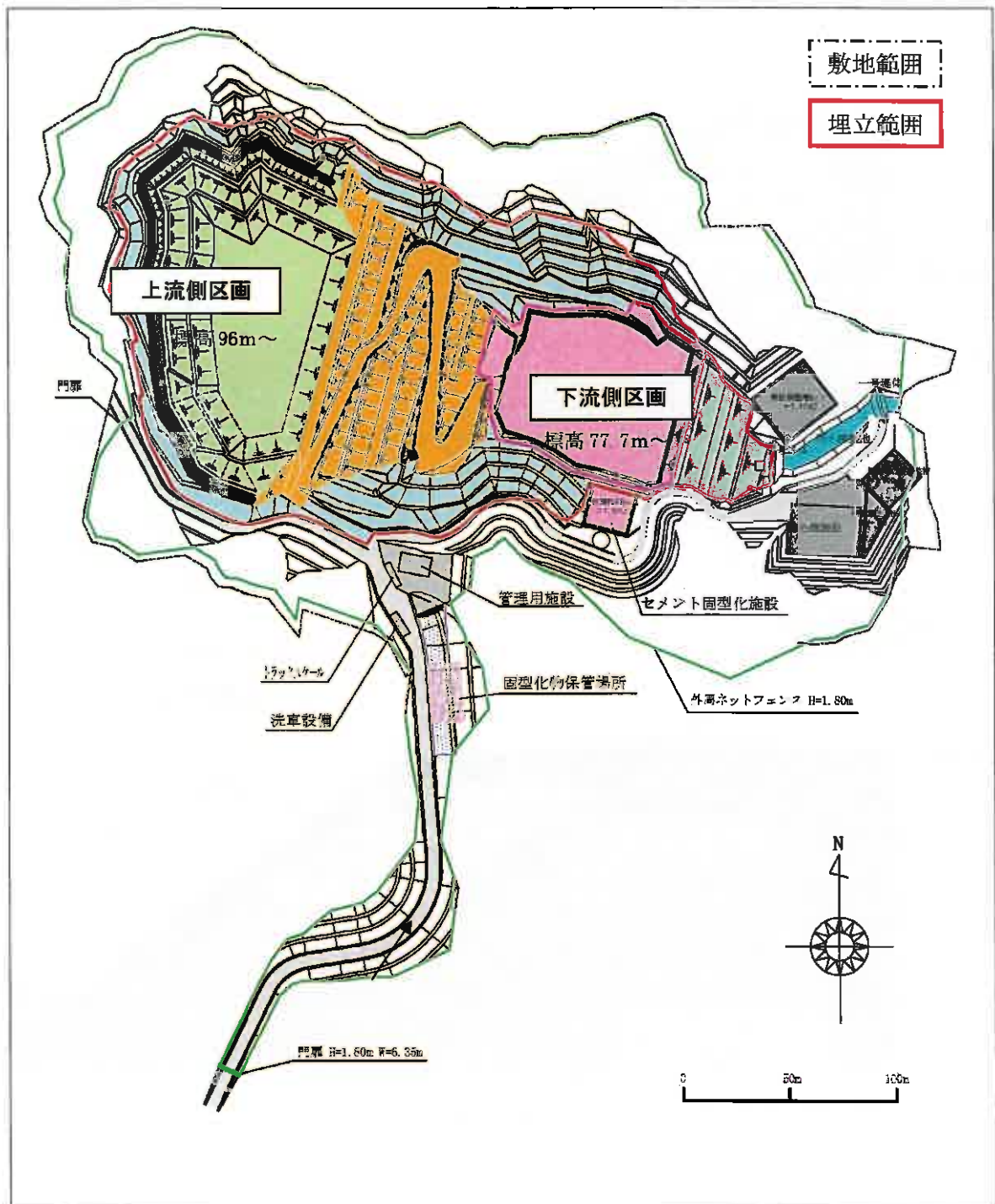
図 1-5(1) フクシマエコテッククリーンセンターの計画図 (埋立開始時)
