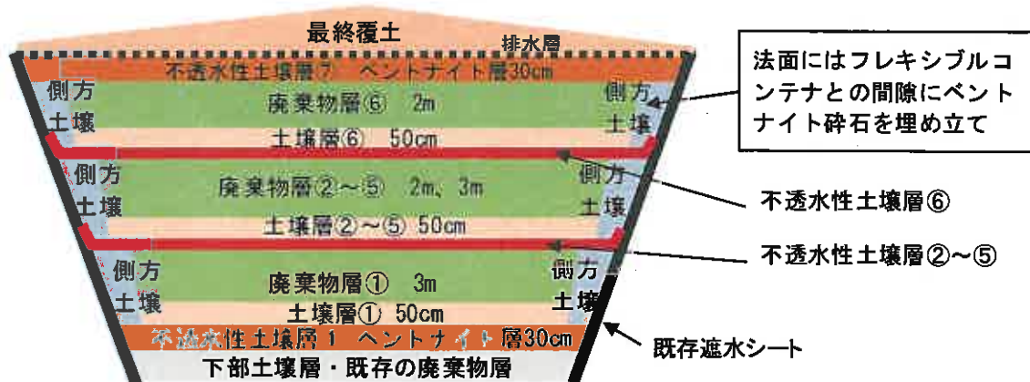
図 2-7(1) セメント固型化した廃棄物の埋立層
