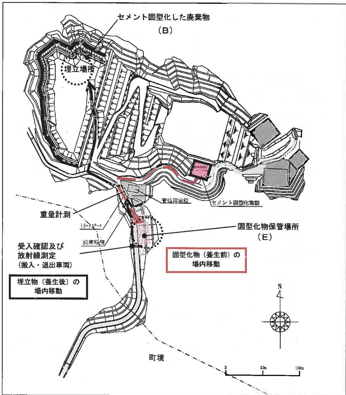
図 2-2(2) セメント固型化廃棄物の場内移動
