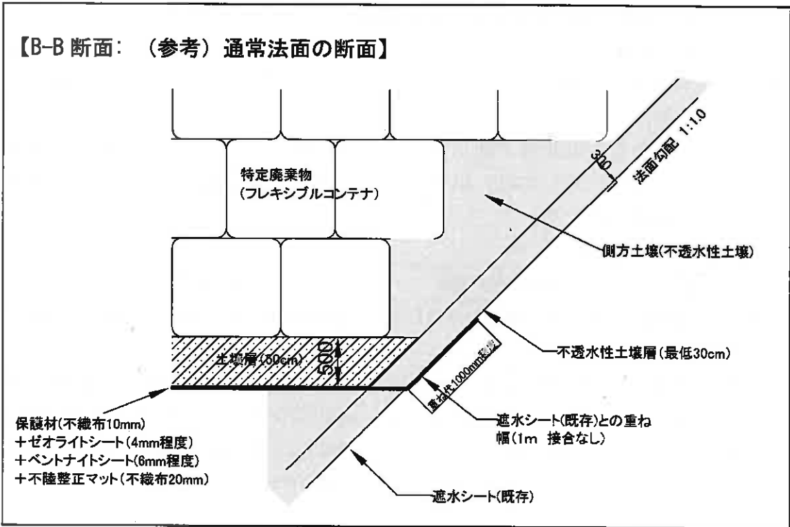
図 2-16(2) (参考) ガス抜き管のない法面の標準構造
