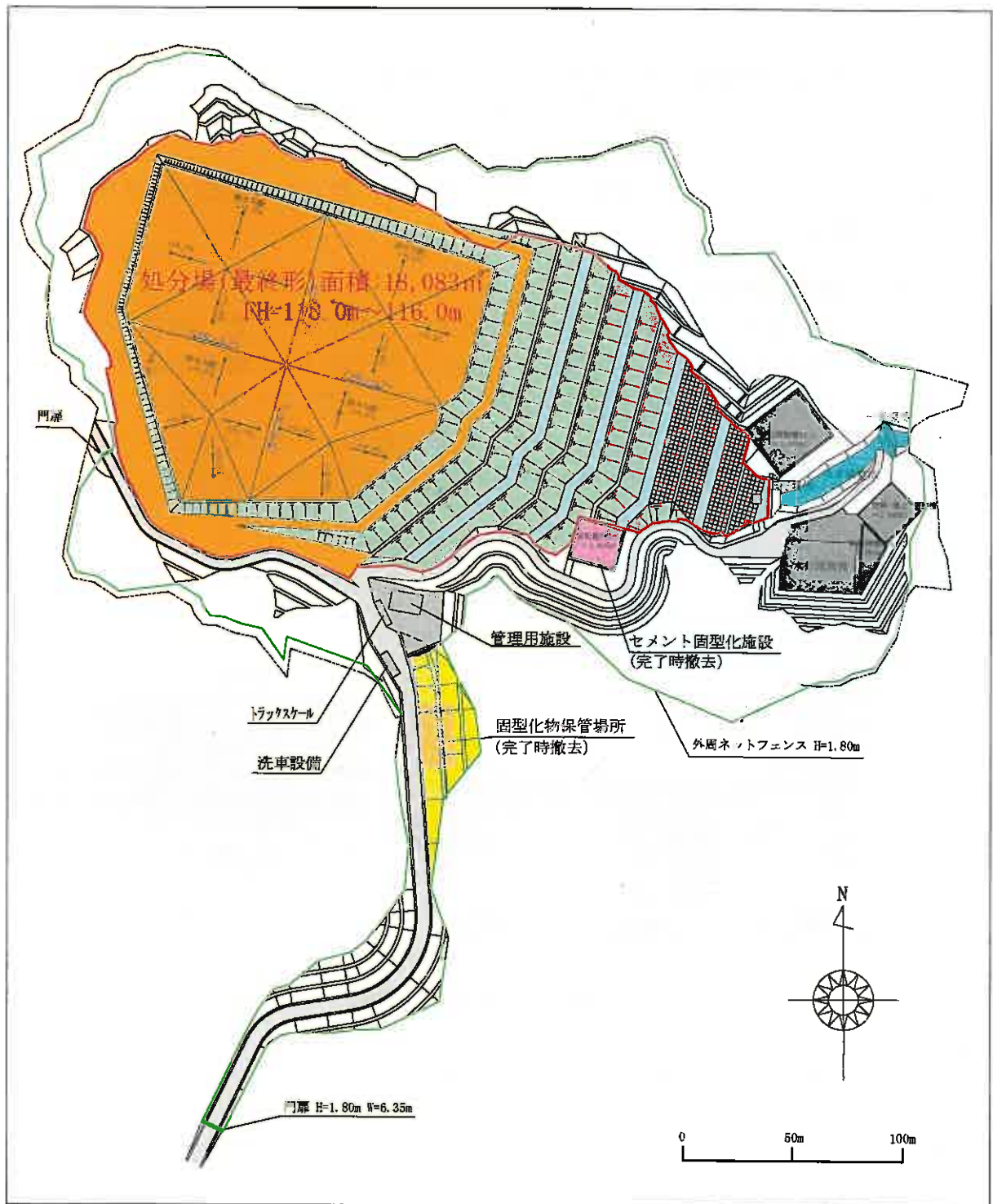
図 1-5(2) フクシマエコテッククリーンセンターの計画図(埋立完了後)
