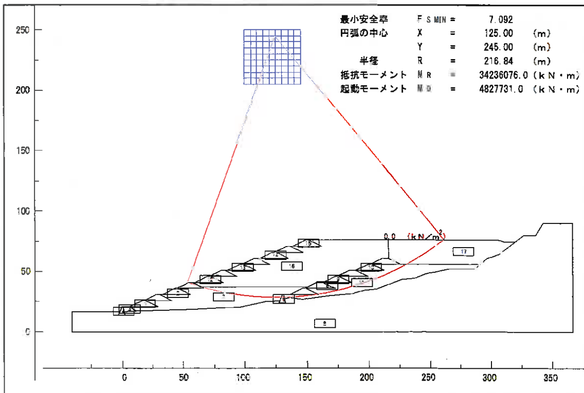
図 2-6 (2) 深いすべり面 (セメント固型化した廃棄物層)
