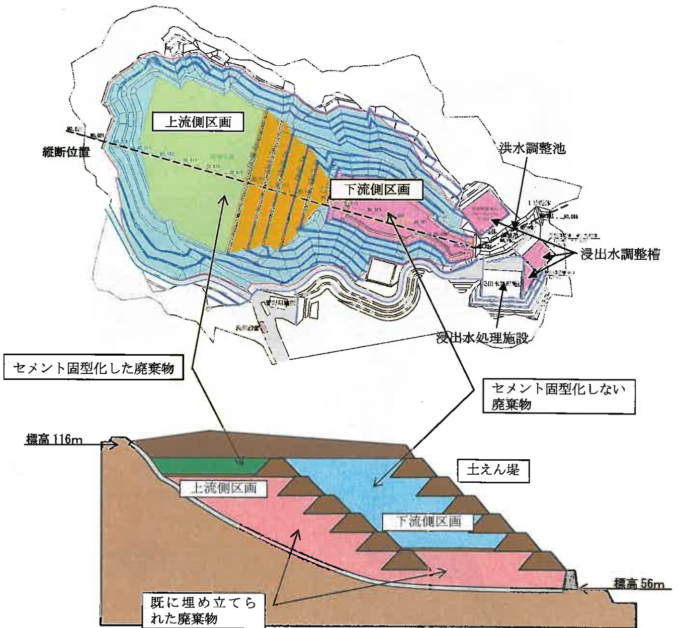
図 1-4 埋立区画概念図
