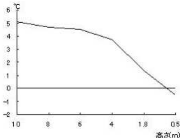
図4 逆転層の出現状況(小松1994)
