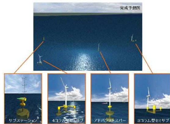
福島県沖における浮体式 洋上windファーム 実証研究事業の完成予定図 (丸紅(株)提供)
