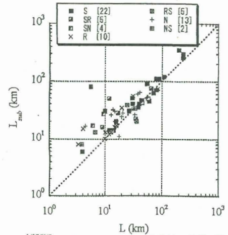
L (地表断層長さ) と L_{hyp} (震源断層長さ) の関係。記号はすべりタイプ別 (S, R, Nはそれぞれ横ずれ断層、逆断層、正断層; SR, SN, RSは横ずれ、縦ずれ、および正断層の混合すべり)を示す。String et al.(2002) (13) によるコンパイルデータのうち、Lと L_{hyp} が記載された地震で、Mwの信頼性が低いと考えられるものを除いた61地震をプロットしている。野澤(2006) (14) より引用。
