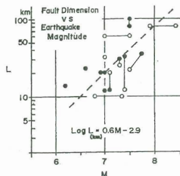
活断層から発生する地震の規模と周期について 松田時彦, 地震 第2輯 第28巻 (1975)より
