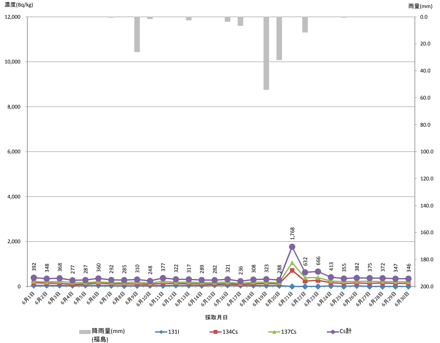
下水道終末処理場放射性物質濃度モニタリング結果 (県北浄化センター) 脱水汚泥 (H24.7月)
