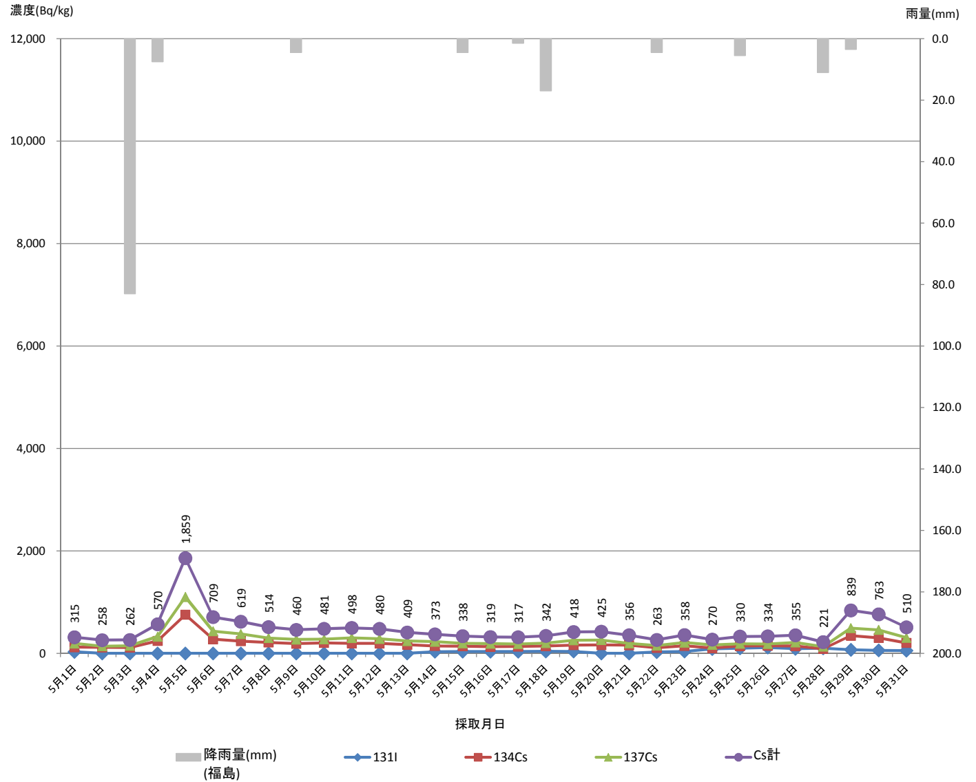
下水道終末処理場放射性物質濃度モニタリング結果 (県北浄化センター) 脱水汚泥 (H24.6月)
