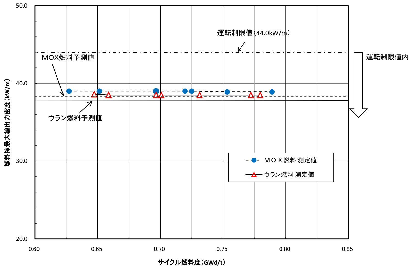
図2 燃料棒最大線出力密度の推移
