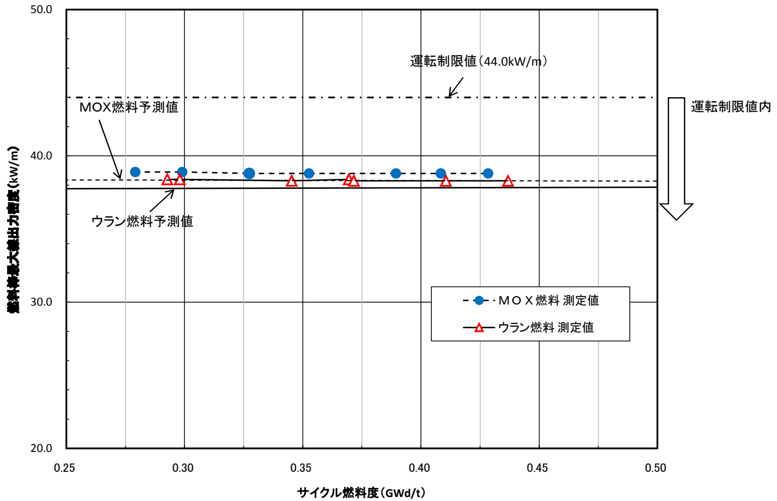
図2 燃料棒最大線出力密度の推移
