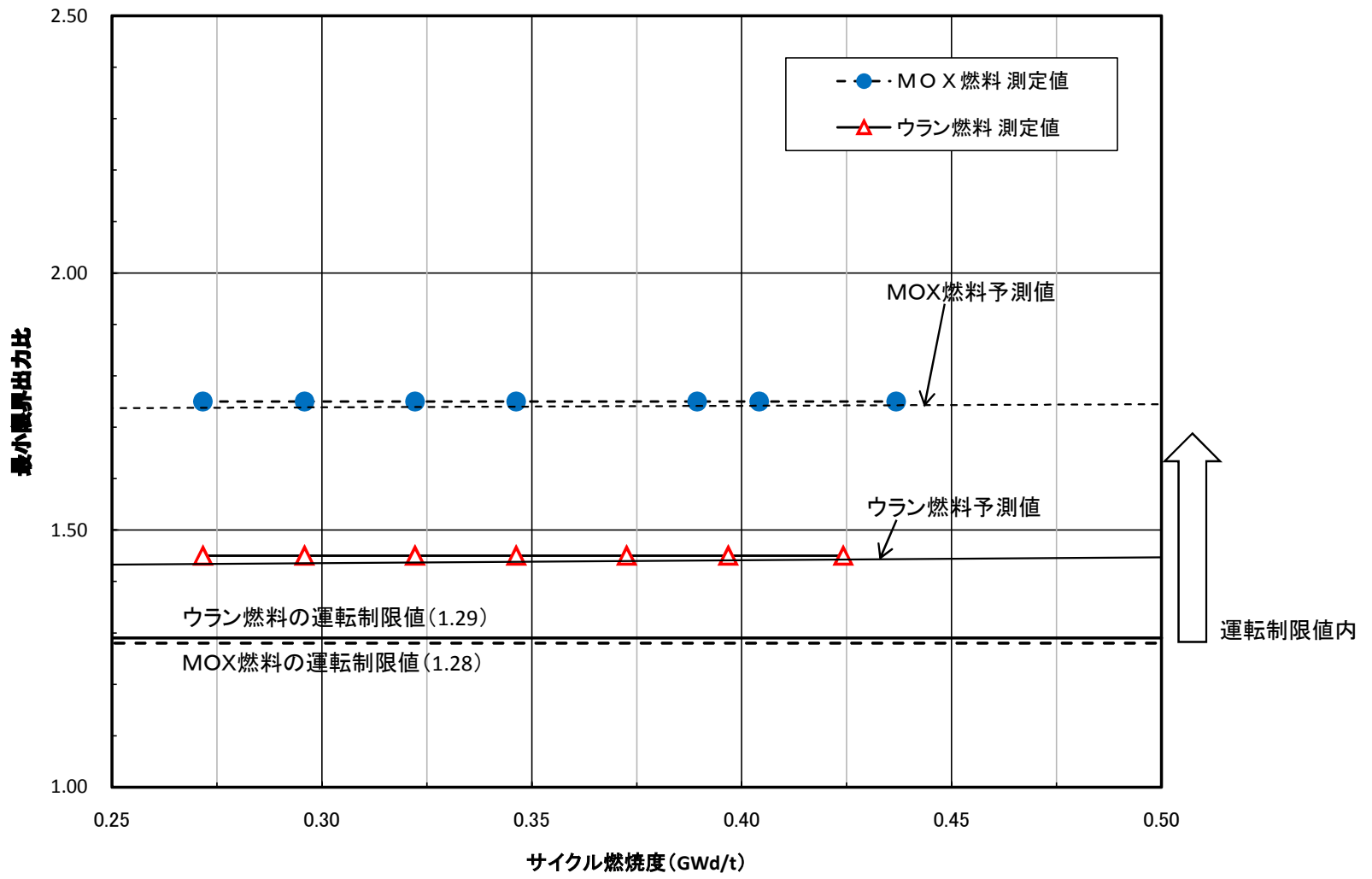
図1 最小限界出力比の推移
