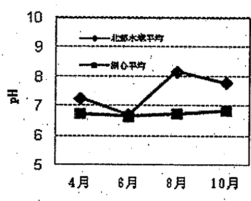
30 図3 北部水域と湖心との比較
