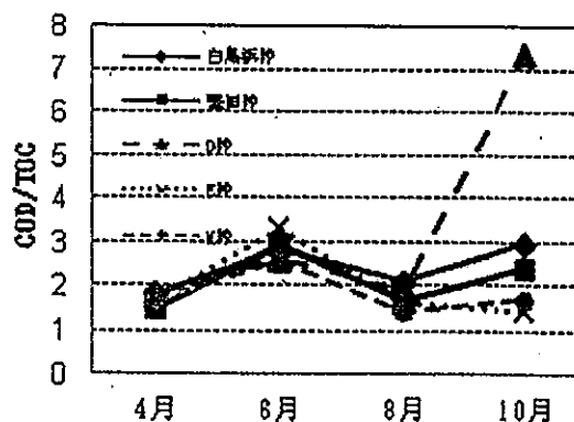
28 図8 COD/TOC比の推移
