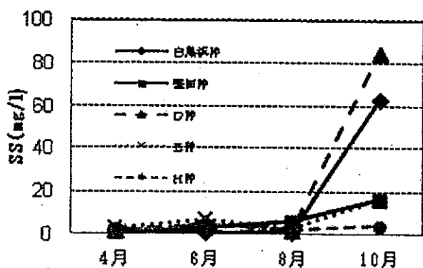
25 図5 SSの推移
