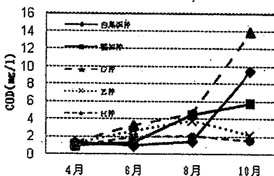
26 図6 CODの推移
