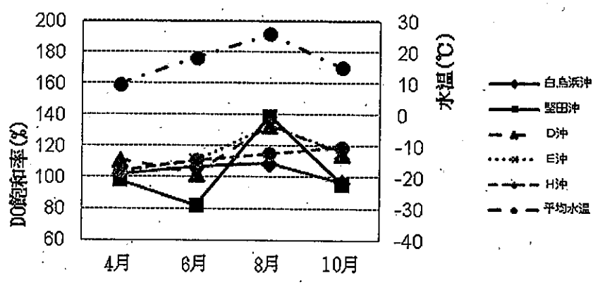
41 図4 DO飽和率の推移
