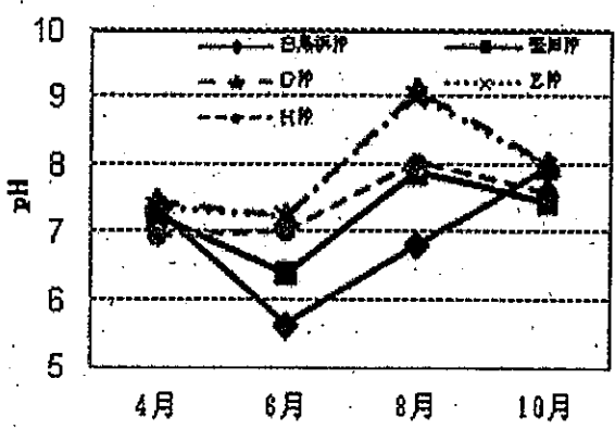
29 図2 北部水域におけるpHの推移
