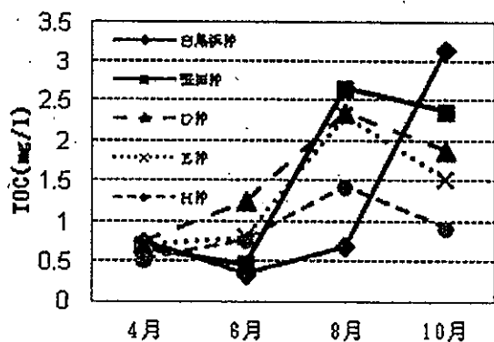
27 図7 TOCの推移
