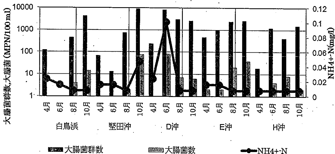
34 図11 大腸菌群数および大腸菌数の推移
