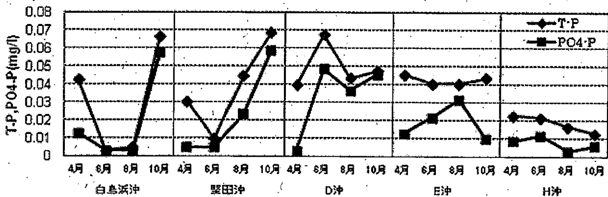
14 15 16 17 18 19 20 21 22 23 図9 T-PおよびPO 4 -Pの推移
