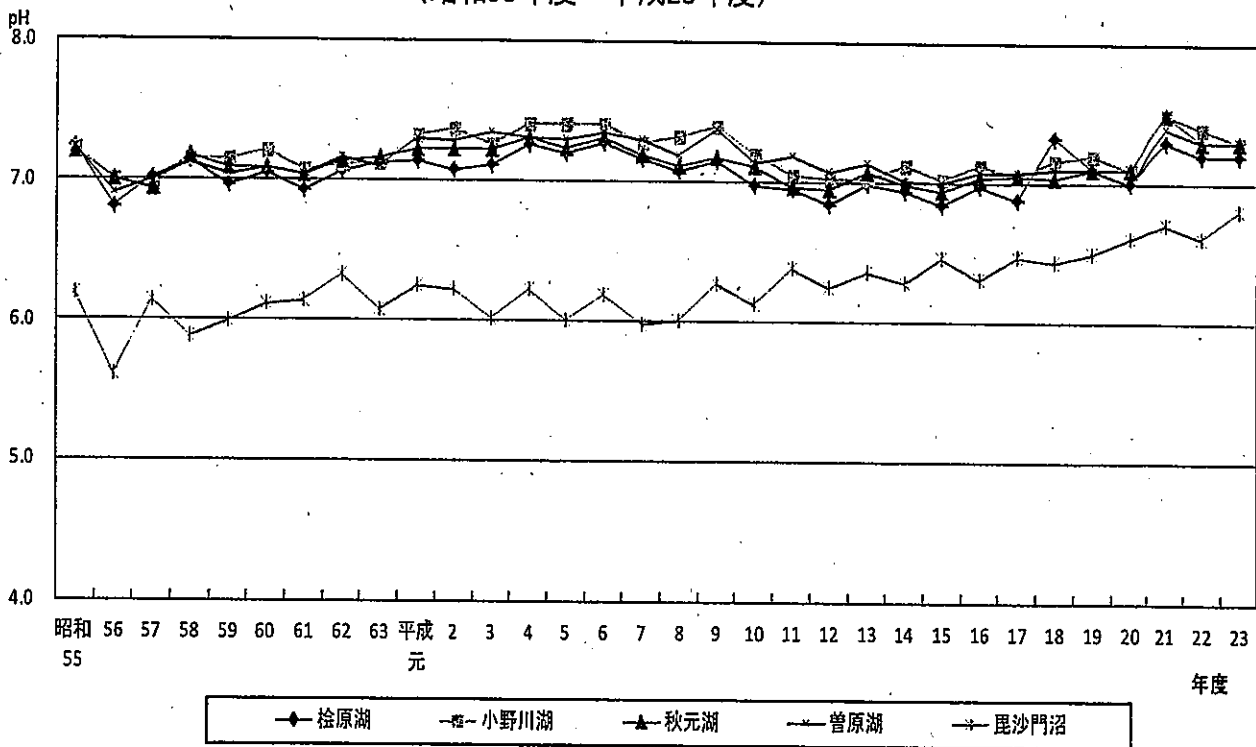
裏磐梯湖沼のpH (湖心全層年間平均)の経年変化 (昭和55年度～平成23年度)
