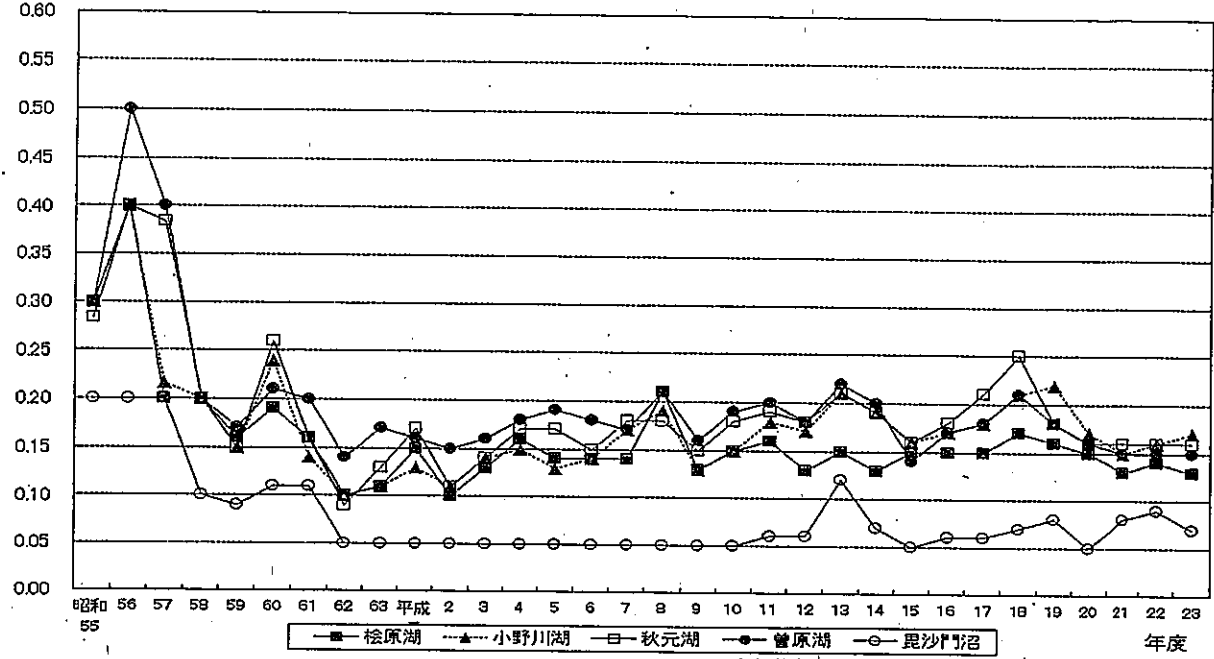
裏磐梯湖沼の全窒素(表層年間平均)の経年変化 (昭和55年度～平成23年度)
