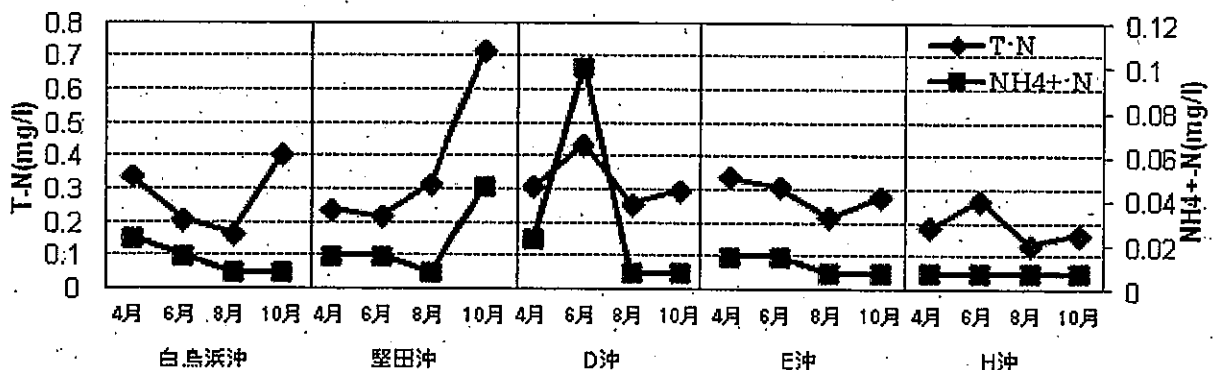
24 25 26 27 28 29 30 31 32 33 図10 T-NおよびNH 4 + -Nの推移
