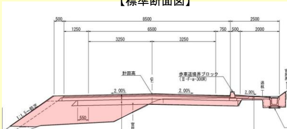
【標準断面図】
