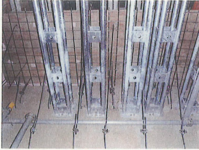
鋼製支柱設置状況
