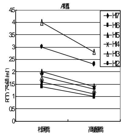
図1-1 BODの縦断分布図
