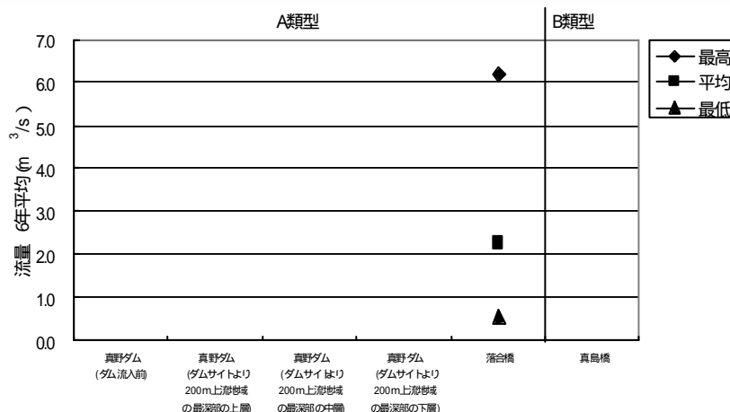
図4-4 流量の縦断分布
