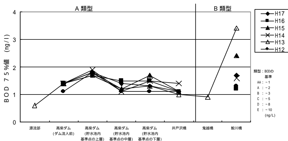
図14-1 BODの縦断分布図
