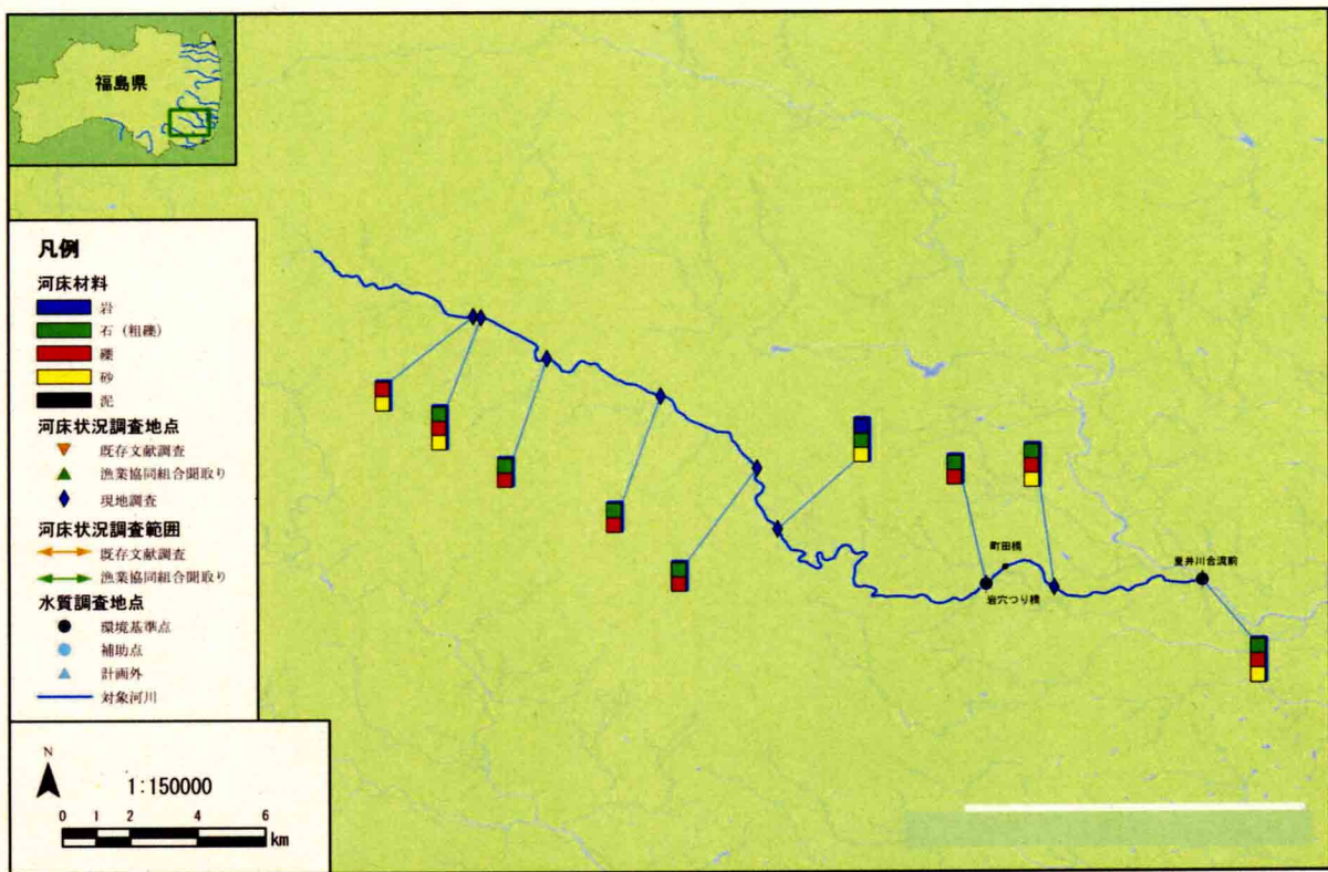
図 12-B 河床材料 (好間川)
