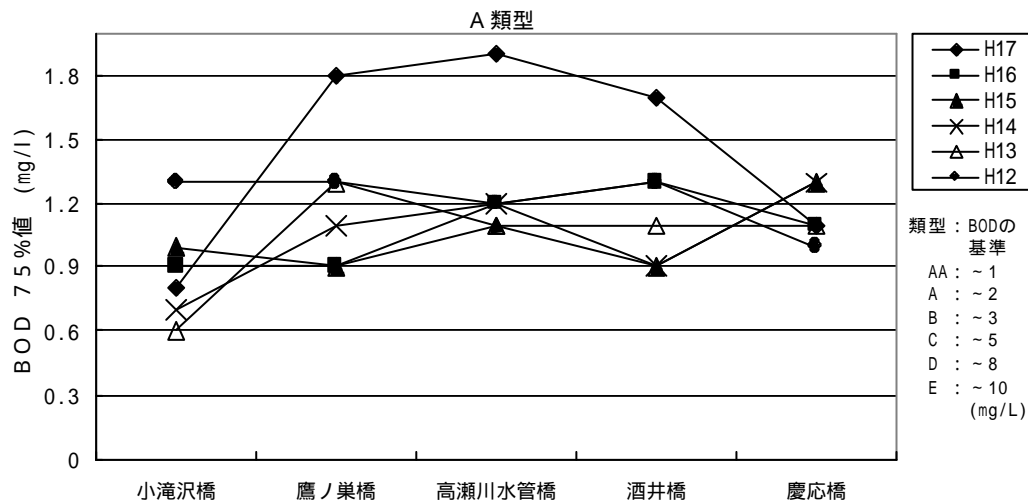
図7-1 BODの縦断分布図
