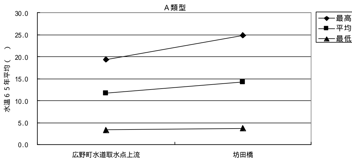
図9-3 水温の縦断分布
