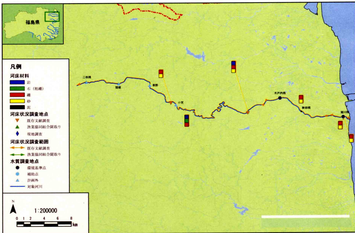
図5-B 河床材料（新田川）
