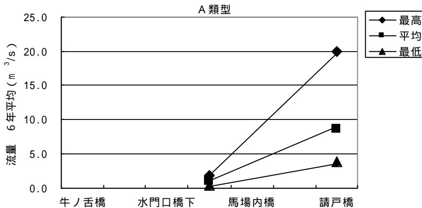
図6-4 流量の縦断分布図
